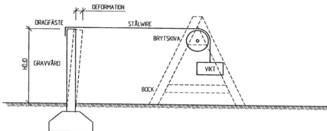
Figur 2. Skiss på konstruktion för statisk provning, elevation 1:20.
