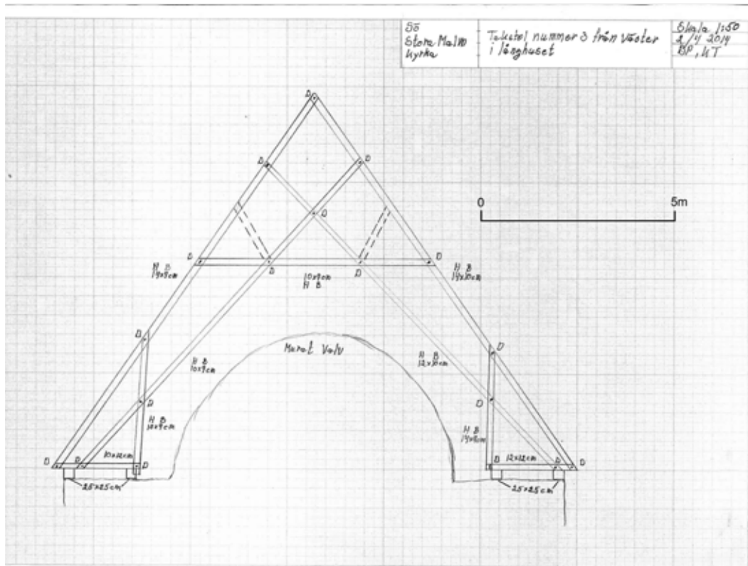
162 Skissuppmätning av takstol i långhuset (SLM D2015-xx).
