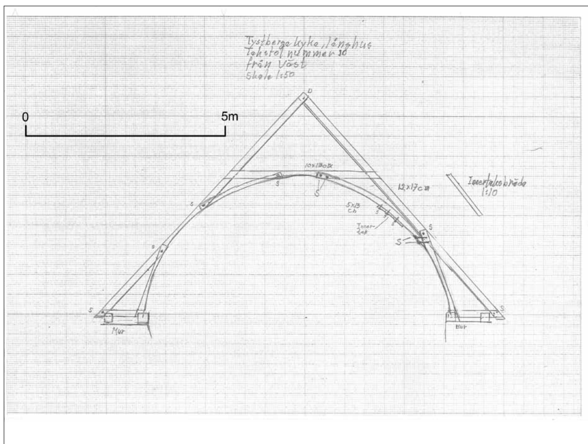
196 Skissuppmätning av tunnvalvstakstol över östra delen av långhuset. BYT MOT NY??
