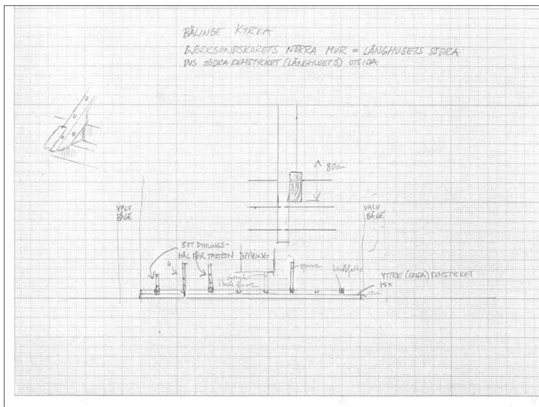
26 Detaljskiss av yttre murremnen vid långhusets södra mur, sett från Björksundskörets vind.
