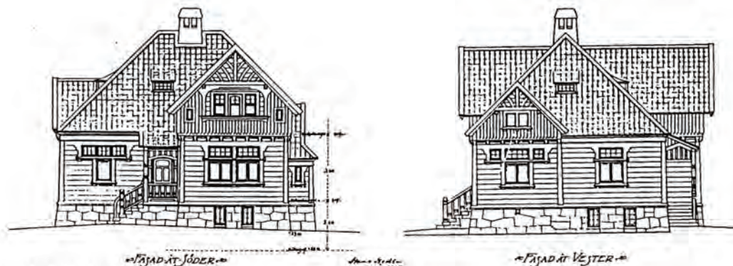
Figur 007. Ritningar över inspektorsbostället som uppfördes 1905, arkitekten var Hans Hedlund. Byggnaden revs 1982. Byggnaden låg tidigare i kv. L.
