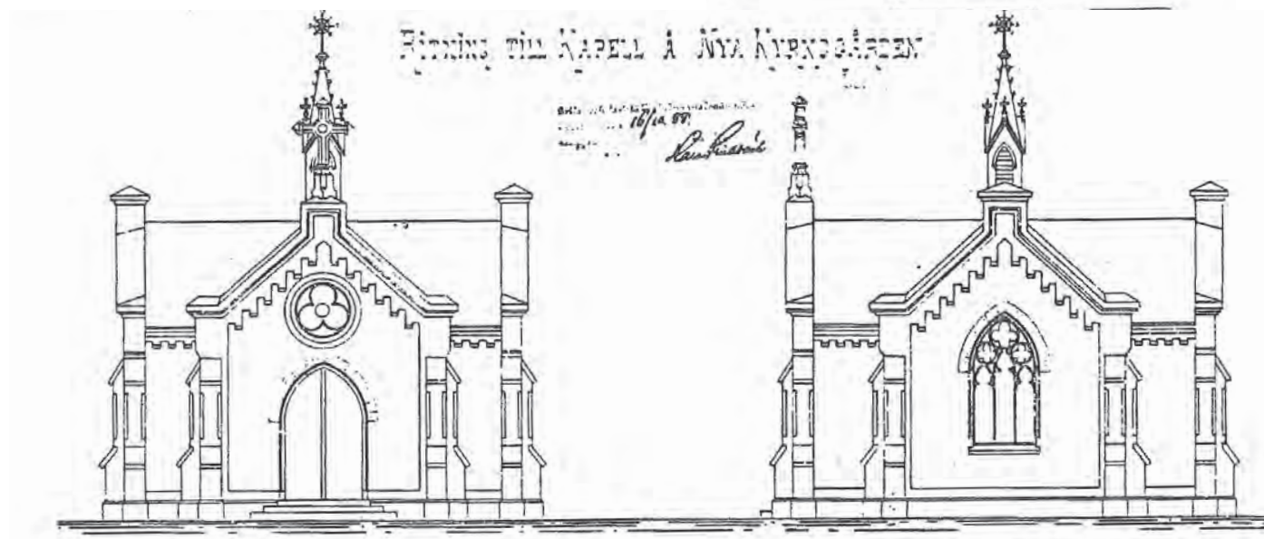
Figur 003. Det ursprungliga kapellet beläget i kvarter K. Revs när S:t Matteus kapell uppfördes 1908.
