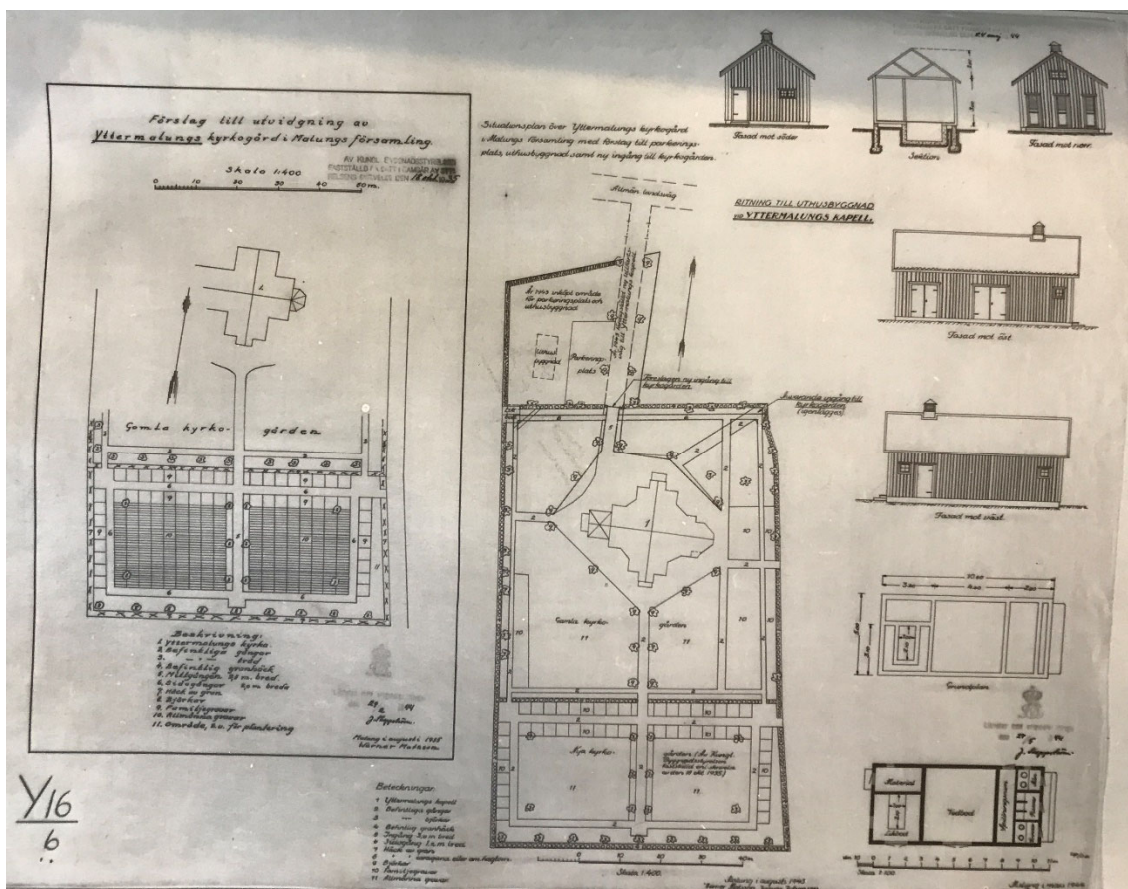
Ritning över kyrkogårdsutvidgning, ny entréväg och uthus, 1935-1944, Werner Matsson. ATA.
