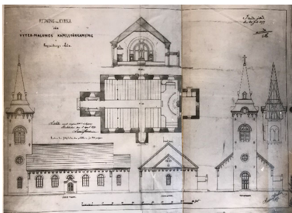
Ritning på kapellet, 1887, ATA.
