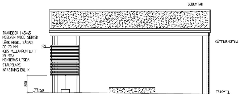
FASAD MOT NORDVÄST
