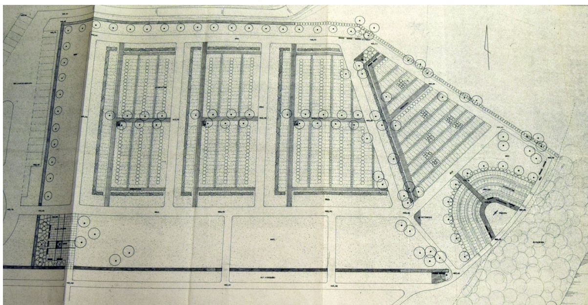
Förslag till utvidgning, 14.07.1967 Edvard Jacobson. Avfotograferad och något beskuren ritning, Värmlandsarkiv.
