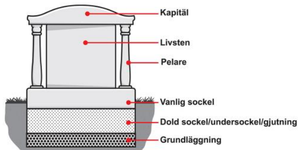
Bild 1, En gravvårds olika delar. Källa: CGK:s Montering och provning av gravvårdar, 2019 Pelare benämns även som kolonn i dagligt tal.
