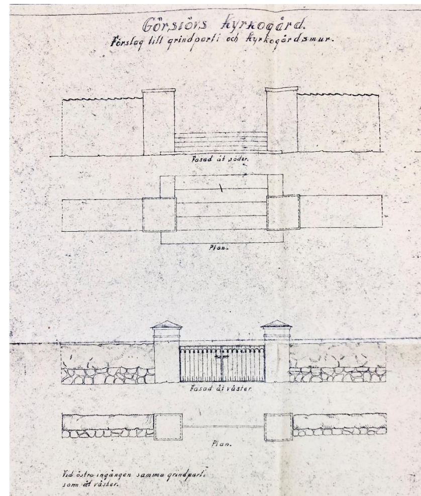
Ritning över grindar och grindstolpar till den nya delen och en ny öppning i den gamla muren med grindpelare och trappa upp till den äldre delen av kyrkogården. Vem som ritat och när är tyvärr oklart. Källa: kyrkoarkivet.
