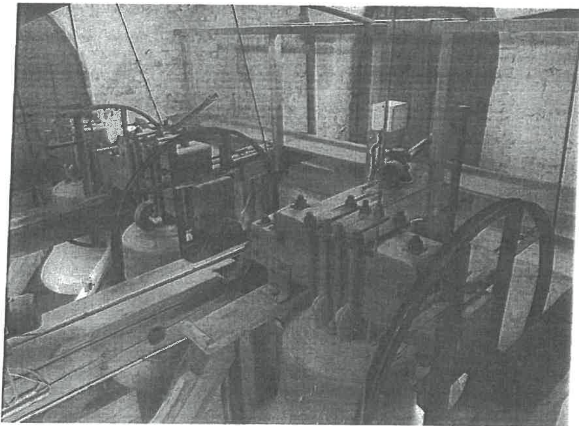
Vy över klockbocken och de tre kyrkklockorna.
