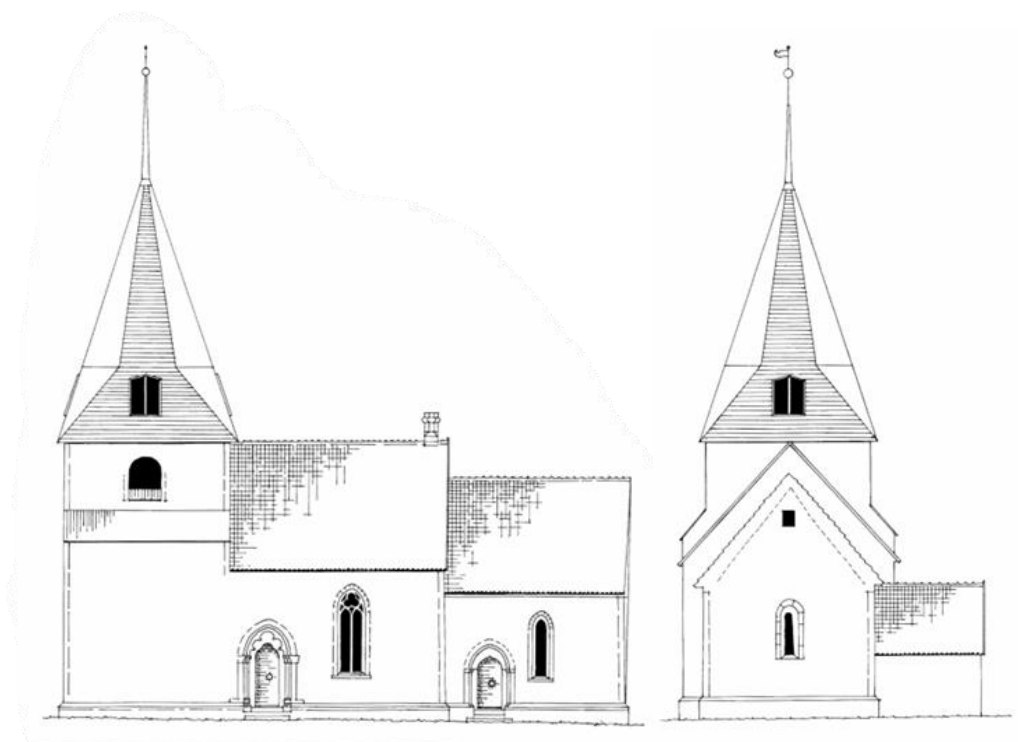
Fasader mot söder och öster. Uppmätning Gunnar Redelius 1998. Efter Sveriges Kyrkor 224, Gotland IX:1 (1998).
