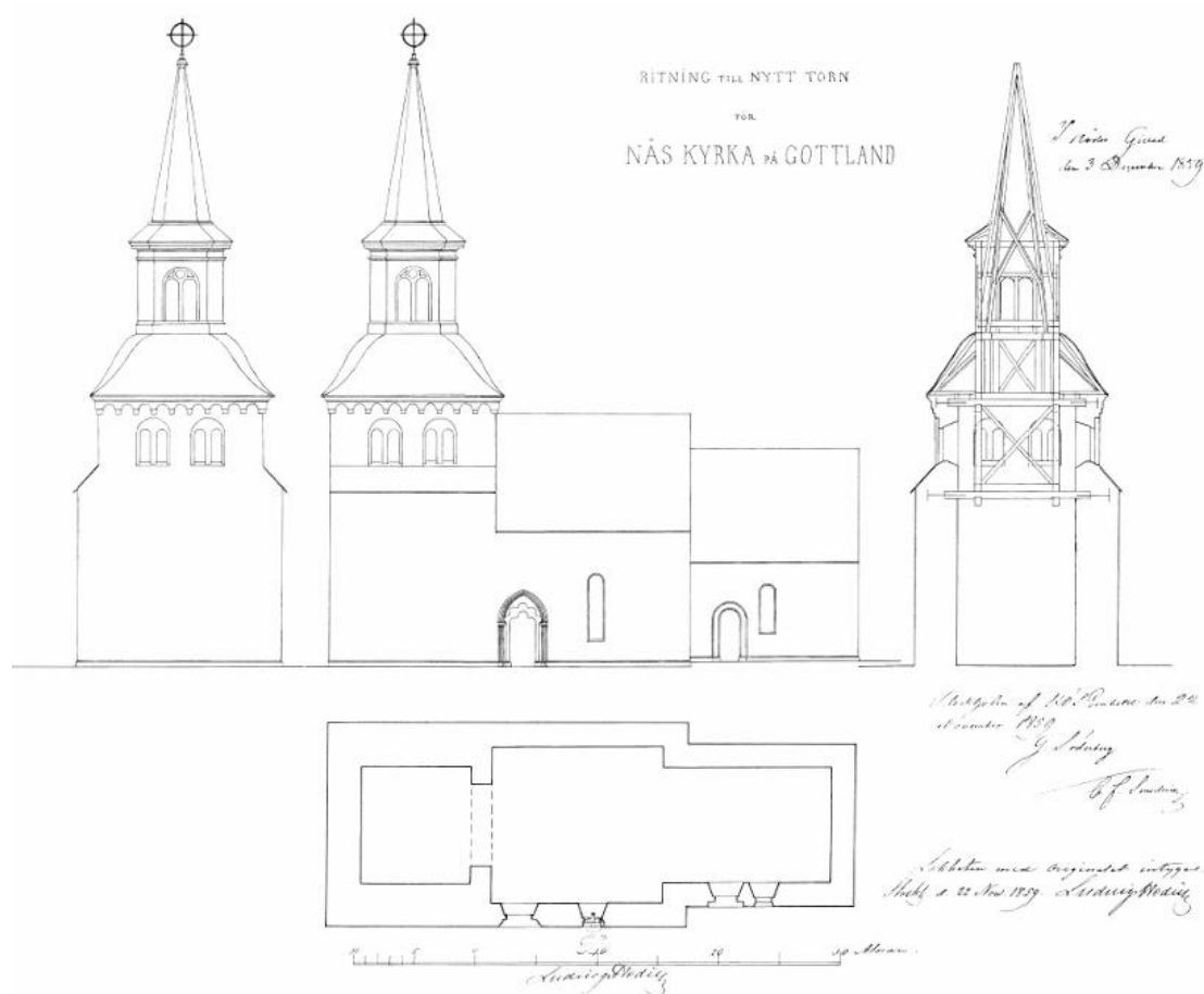
Ritning av Ludvig Hedin 1859 som bearbetning av Klingwalls förslag. Gillad av Kungl. Maj:t men ej följd. Efter Sveriges Kyrkor 224, Gotland IX:1 (1998).
