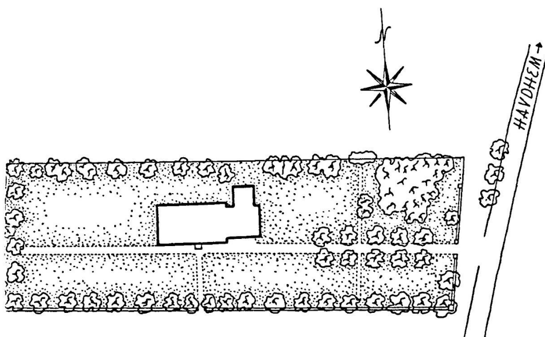
Situationsplan Näs kyrka och kyrkogård. Uppmätning av J Söderberg 1943. Ur Vård och underhållsplan 2010.
