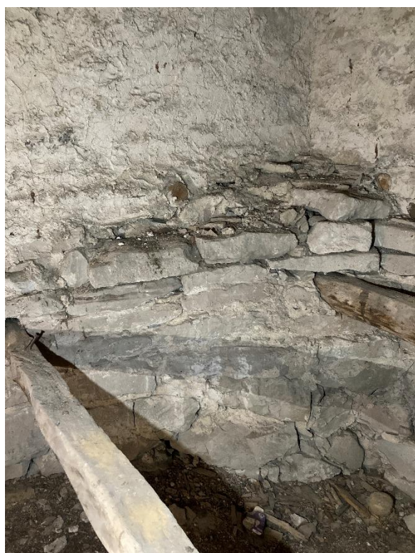
Tornets första övervåning. Utbuktning av det äldre murverket i sydvästra hörnet, till synes ursprunglig och utan motsvarighet i de andra hörnen, möjligen ett förberedande för en tänkt murtrappa upp till tornets planerade övervåningar. Till höger en av bjälkarna tvärs över rummet med synliga urtag, troligen från tornets tidigare träöverbyggnad. Foto JL 2025.
