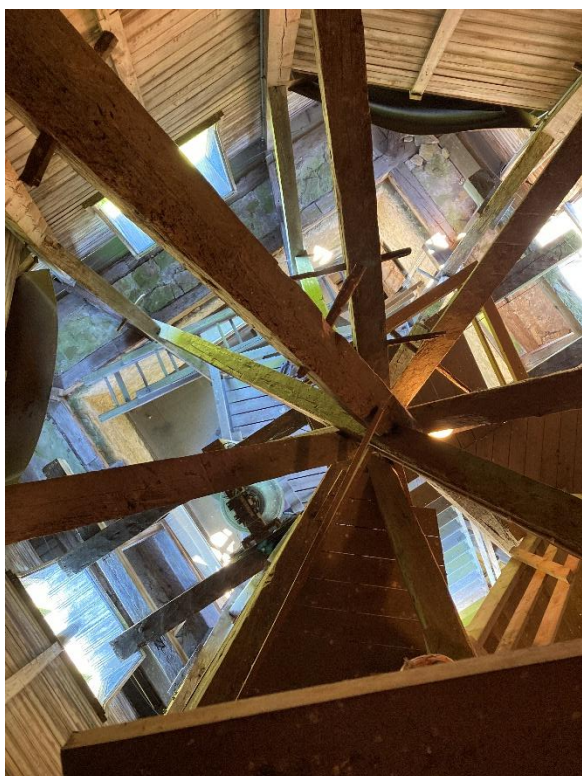
Huvens inre konstruktion sedd rakt ovanifrån och uppåt. Foto JL 2025.
