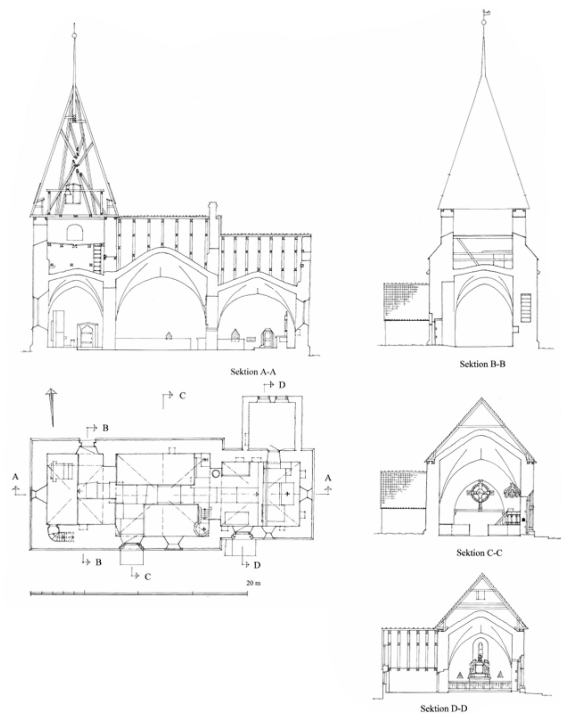
Längdsektion mot norr och plan samt tvärsektioner genom tornet, långhuset och koret mot öster. Uppmätningar John Söderberg 1943, kompletterade av Gunnar Redelius 1998. Efter Sveriges Kyrkor 224, Gotland IX:1 (1998).
