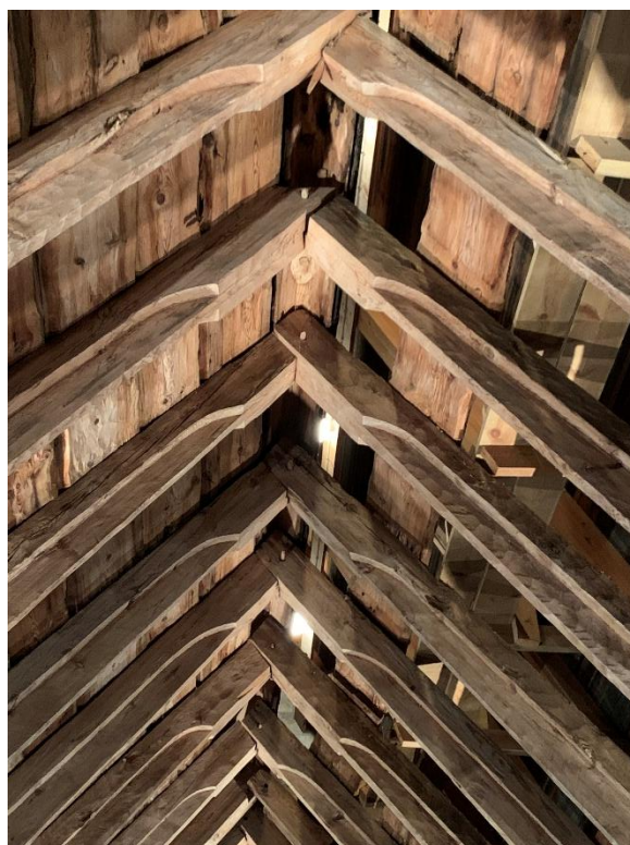
Detaljer av den tidigmedeltida takstolen över långhuset, vars detaljer ursprungligen var synliga från kyrkorummet. Foto JL 2023.
