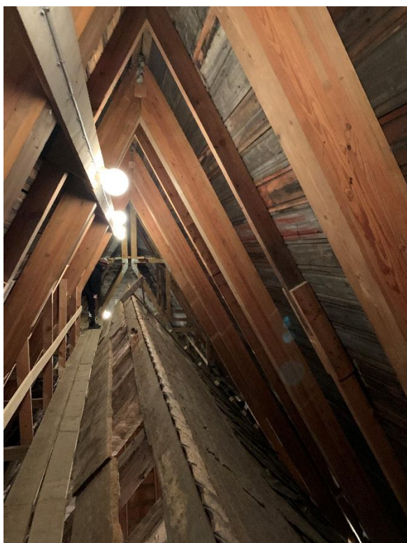
Det tidigmedeltida taket samt över det takstolen från 1960-talet till det nuvarande yttertaket sedda mot öster. Till höger långhusvindens nordvästra hörn med ett stycke av påmurningen i betong från 1960-talet. Foto JL 2023.
