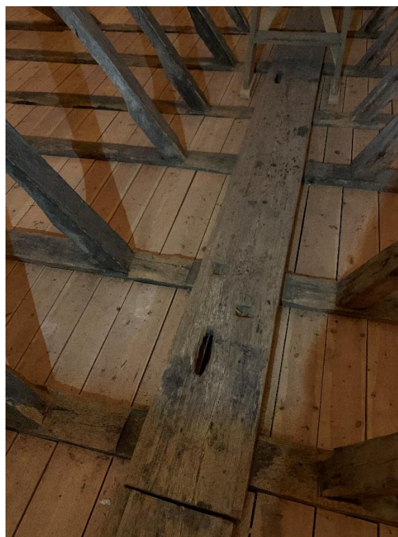
Långhusets takstol sedd mot väster, snett ovanifrån. Till höger styrbrädan, som utgjort brygga mellan tornet och korvinden när takstolen var öppen. Foto JL 2023.
