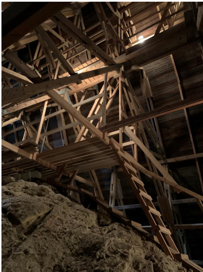
Del av korets takstol och korvinden, sedda mot sydöst. Foto JL 2023.
