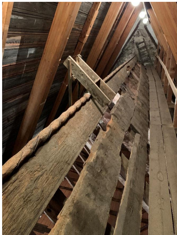
Långhusets tidigmedeltida takstol sedd mot väster. Till höger med del avnockbrädan och underpanel till spånklädseln. Foto JL 2023.
