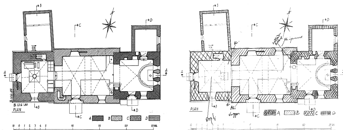
Kyrkans plan. Uppmätning John Söderberg 1943, reviderad 1972. ATA. Byggnadsperioder: A och B 1200-talets andra fjärdedel, C omkring 1300, D 1819-1820 (magasinet) och 1832-1833 (sakristian). Fönstren förstörades respektive upptogs 1835. Av ritningen till höger framgår utseendet före restaureringen 1969-1971 med fönster i långhusets norra mur, orgel mitt i ringkammaren och dopfunten på triumfbågens norra sida.
