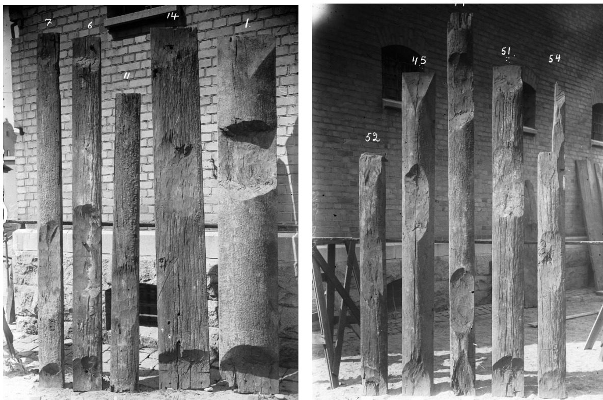
Delar av en äldre träkyrka, påträffade som golvplankor 1916 och lösgjorda. Nu på SHM. Foto Harald Faith-Ell 1925, ATA.
