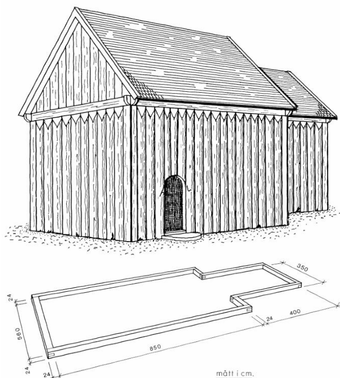
Rekonstruktion av den tidigare träkyrkan utifrån de påträffade delarna. Erland Lagerlöf och John Söderberg 1973. Efter Sveriges Kyrkor 156, Gotland VI:6 (1974). Till höger plankor med bevarade rester av väggmålning. Nu på SHM. Foto JL 2025.
