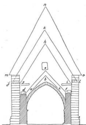
Schematisk skiss av tvärsnittet öster om långhusets östgavel mot väster.
