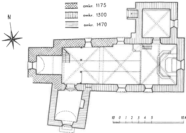
Sånga kyrkas plan.
