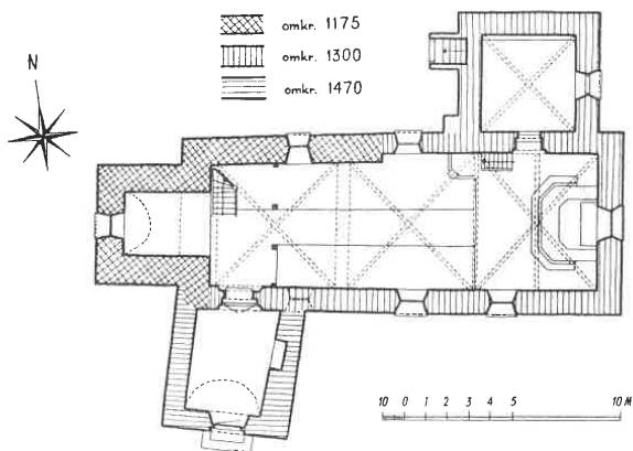
Sånga kyrkas plan. Skala 1:300.
