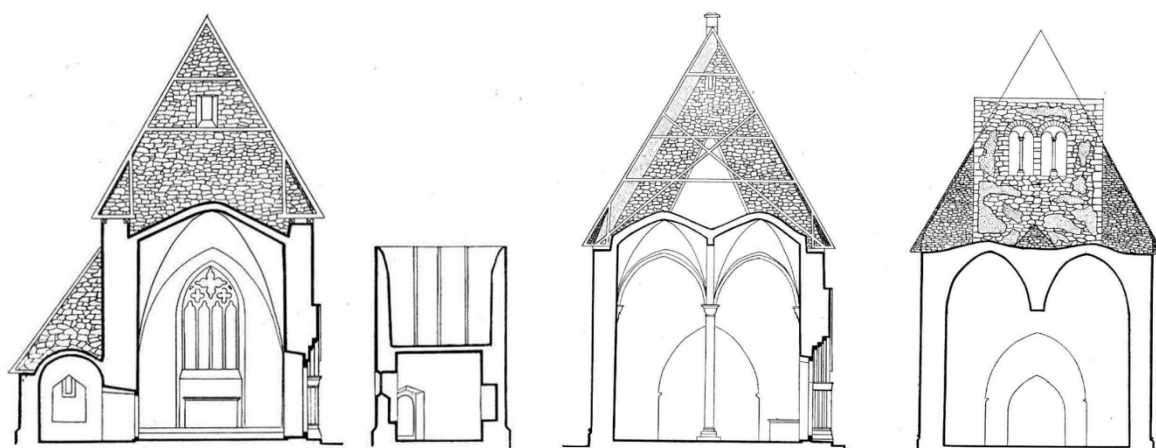
Tvärsektion av koret mot öster och längdsektion av sakristian mot söder. Uppmätning från 1940-talet. Efter Sveriges Kyrkor, Gotland IV:1, volym 61.
