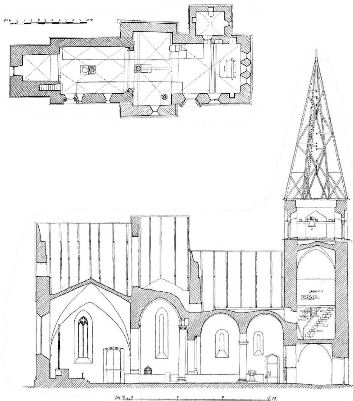
Plan och längdsektion mot söder. Byggnadsperioderna i planen avser: krysskafferat, 1200-talets början och snedskafferat 1200-talets slut. Vid restaureringen 1957 avlägsnades väggen för ringkammaren, orgelharmoniet vid den östra kolonnen samt kaminen. Sakristian byggdes till åt väster med en trappa till ett pannrum i en nybyggd källare. I sektionen saknas murtrappans mynning i första våningens sydvästra hörn, södra ljudgluggens bågar samt skorstenen. Uppmätningar av Sten Wennerström och Adolf Niklasson 1921. Efter Sveriges Kyrkor (volym 42), Gotland band II (1935).
