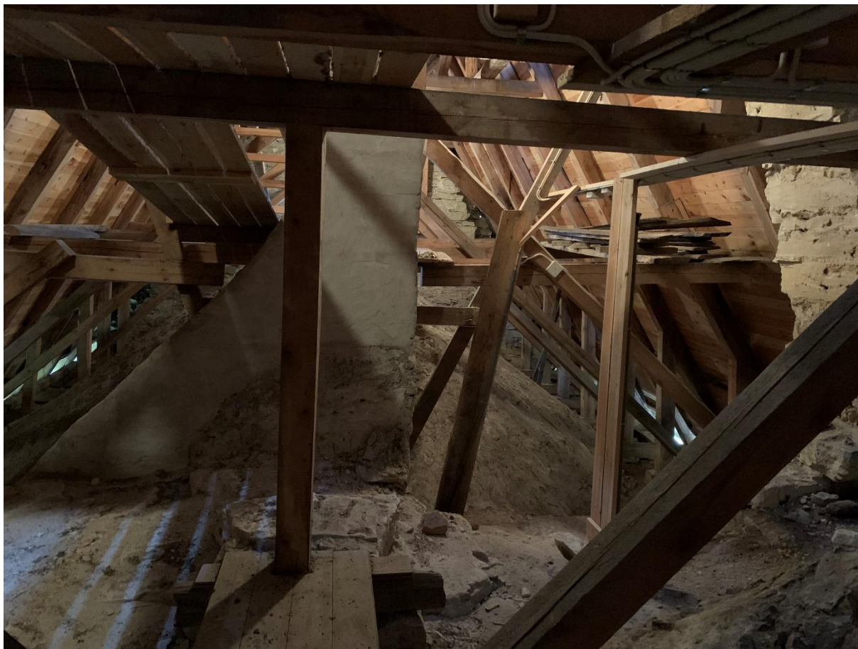
Korvinden mot öster i nivå med valvet. I förgrunden skorstensstocken. Foto JL 2021.
