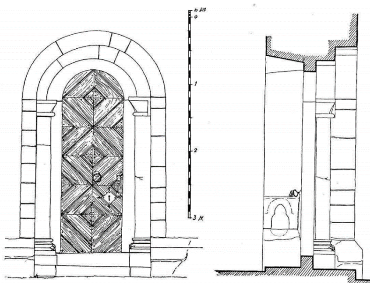
Långhusportalen, 1200-talets början. Foto JL 2021. Elevation och sektion. Uppmätning av Sten Wennerström och Adolf Niklasson 1921. Efter Sveriges Kyrkor (volym 42), Gotland band II (1935).
