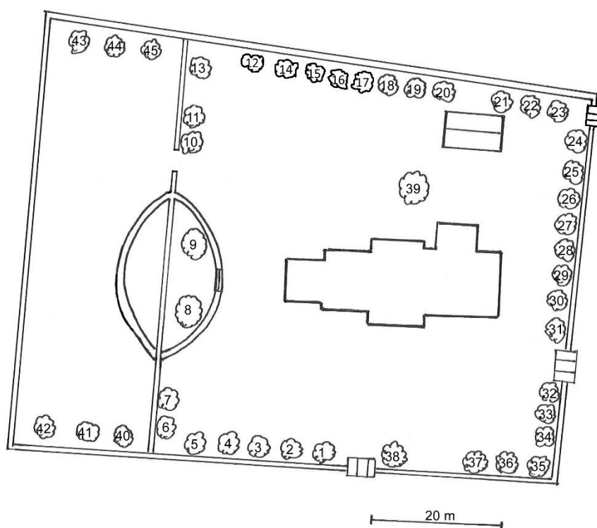
Vallstena kyrka. Situationsplan 2011, reviderad 2021, Gotlands Museum.
