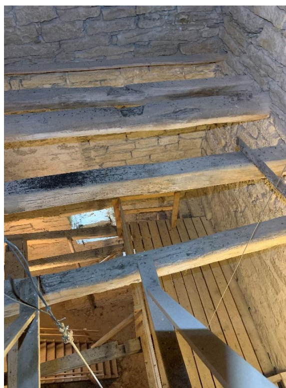
Murtrappa i norra muren från tornets andra övervåning och uppåt, sedd uppifrån mot väster. Vid vilplanet ingång till tornets tidigare tredje övervåning samt ljusglugg i norra muren, något större än de övriga. Till höger bjälklaget till tidigare tredje övervåningen sett nedåt åt sydväst. Två av de till synes ursprungliga bjälkarna har urtag för tidigare anordningar eller för att bjälken tidigare haft annan funktion. Foto JL 2021.
