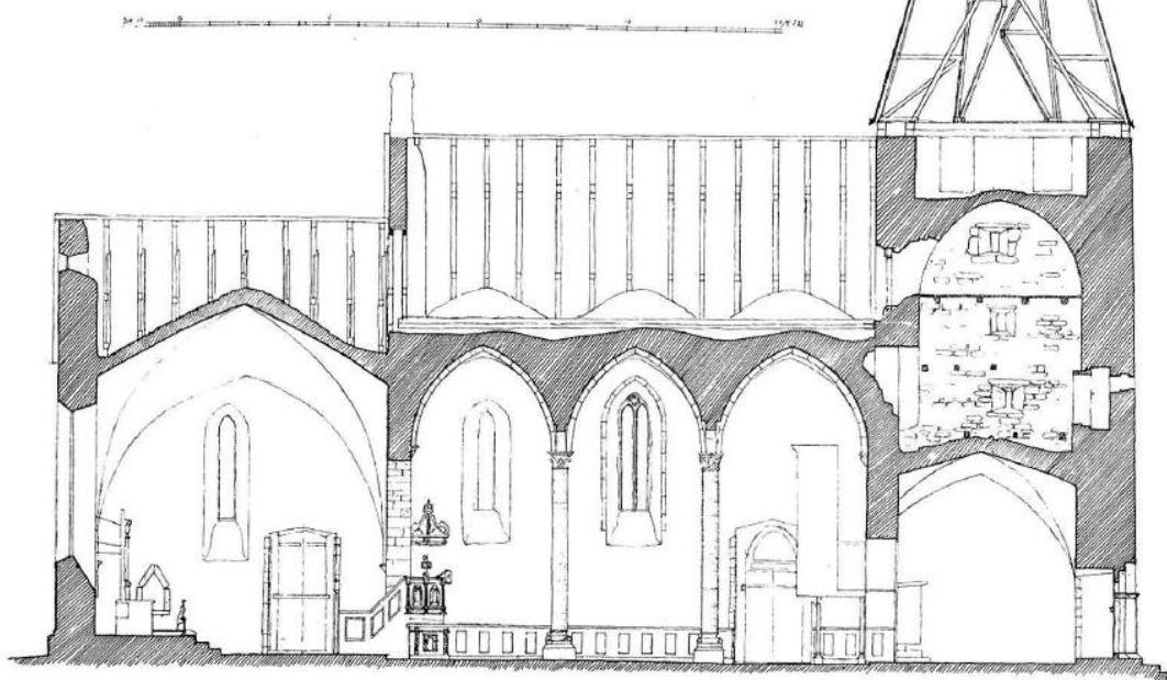
Längdsektion mot söder samt valvplan. Läktaren har senare rivits. Uppmätning Sten Wennerström och Adolf Niklasson 1921. Efter Sveriges Kyrkor volym 42, Gotland band II (1935).
