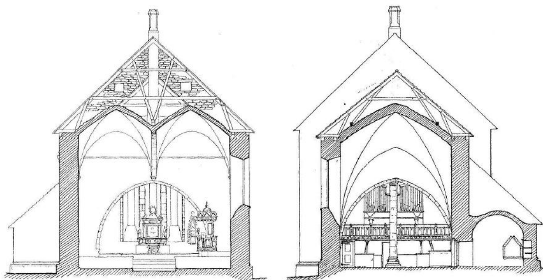
Tvärsektioner genom långhuset mot öster samt koret och sakristian mot väster. Uppmätning Sten Wennerström och Adolf Niklasson 1921. Efter Sveriges Kyrkor volym 42, Gotland band II (1935).
