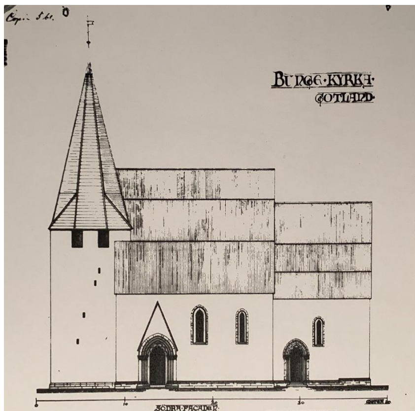
Kyrkans sydfasad med yttertaken ritade efter Laurins ritning från 1853 och strävpelaren slopad. Uppmätning av arkitekten Gustaf Pettersson, troligen ca 1890-95, möjligen tänkt som restaureringsförslag. Original i Överintendentsämbetets arkiv (B 212:4). ATA, K-byråns ritningsfoton.
