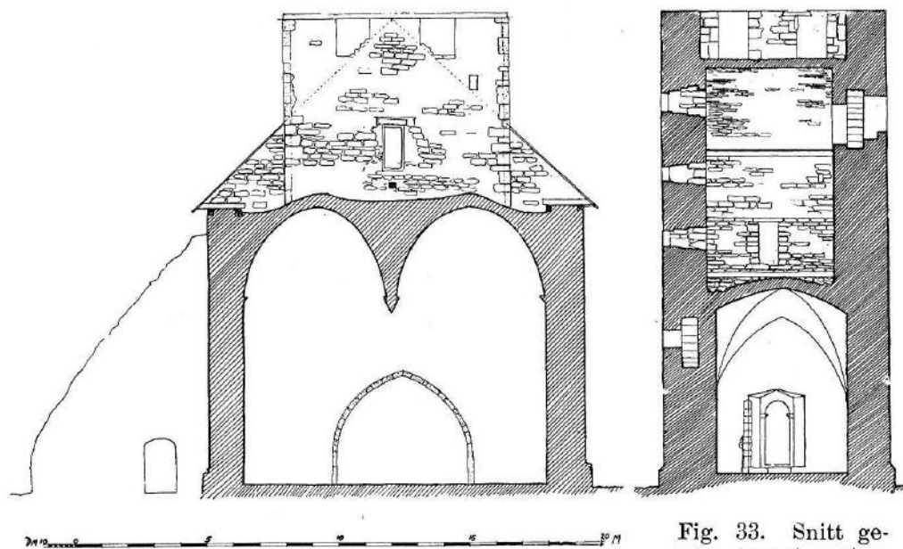
Tvärsektion genom långhuset och tornet mot väster. Uppmätning Sten Wennerström och Adolf Niklasson 1921. Efter Sveriges Kyrkor volym 42, Gotland band II (1935).
