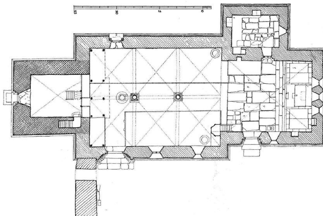
Kyrkans plan. Uppmätning Sten Wennerström och Adolf Niklasson 1921. Efter Sveriges Kyrkor volym 42, Gotland band II (1935). Tornet byggdes vid 1200-talets början, kor och långhus under 1300-talets andra fjärdedel och strävpelaren möjligen på 1700-talet. Senare har läktaren rivits och ringkammaren inretts till mindre kyrkorum.
