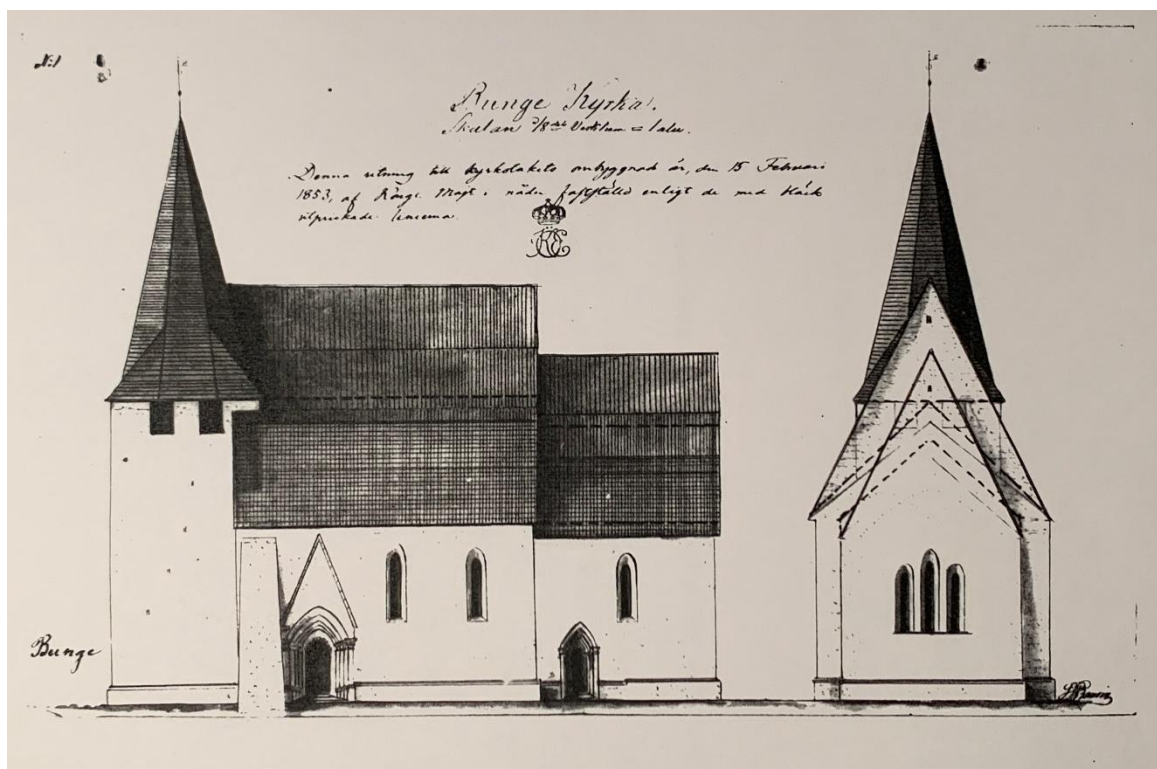
Fasad mot söder och öster, visande de höga takfallen samt förslag till ny, sänkt takvinkel enligt två olika alternativ, där streckad linje anger att korets och långhusets takfot skulle ligga i samma nivå och takfallen ha samma vinkel. Ritning av Carl Philip Laurin, Fårösund, 1853. Original i Överintendentsämbetets arkiv (B 212:1). ATA, K-byråns ritningsfoton.
