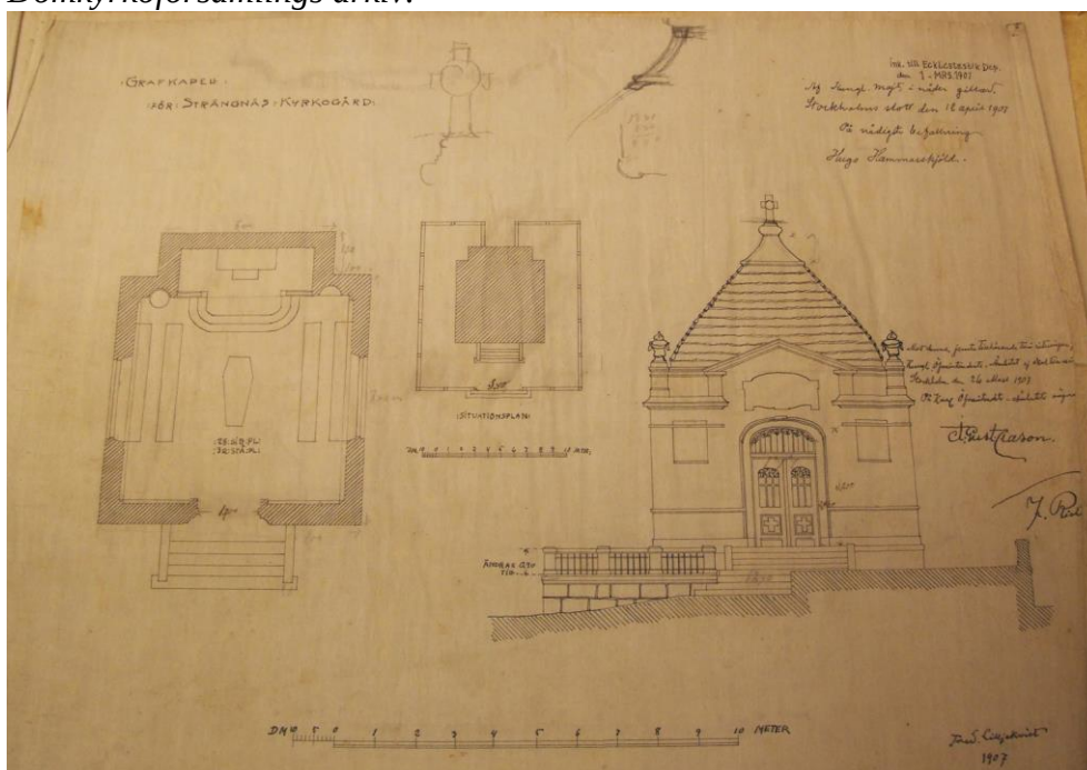
Arkitekt Fredrik Lilljekvists ritning på gravkapell 1907. Strängnäs Domkyrkoförsamlings arkiv.
