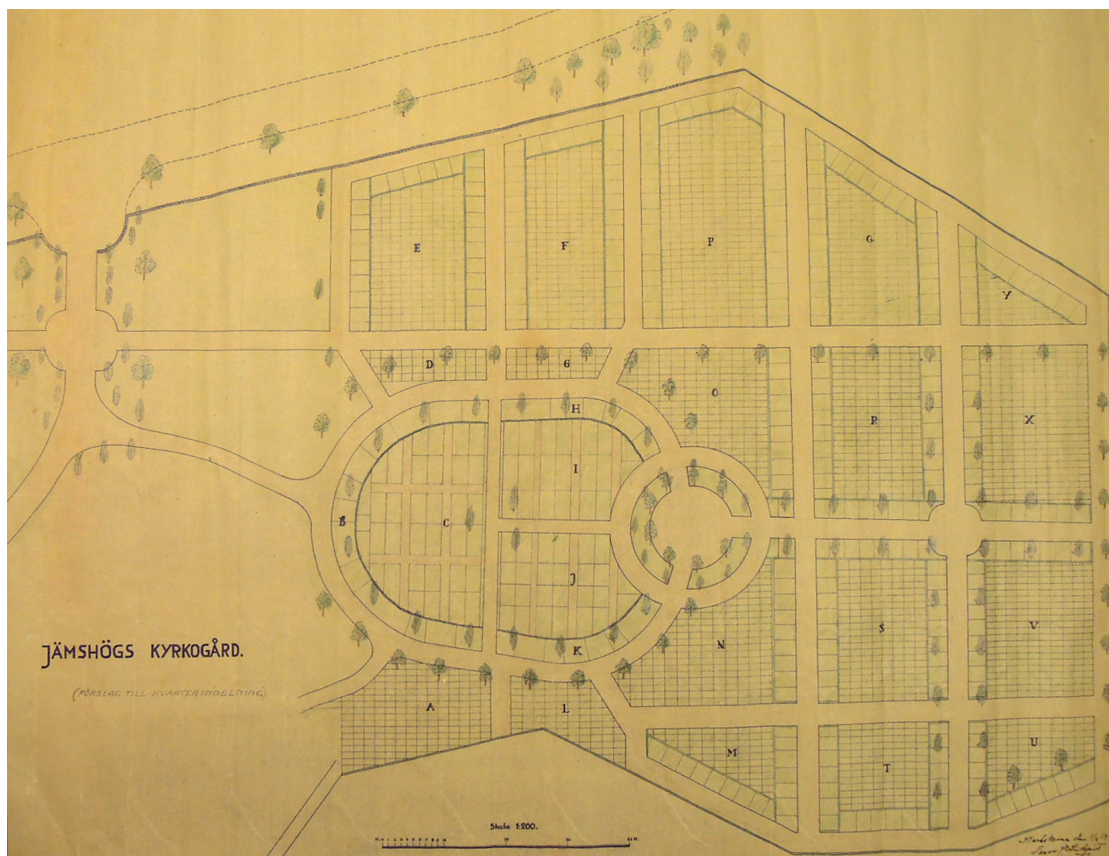
Kyrkogårdsutvidgning mot norr, ritning till kvartersindelning, signerad 1932 av stadsträdgårdsmästaren i Karlskrona Paavo J. Lindqvist. Även utvidgningarna från 1901 och 1914 återges. (Jämshögs kyrkoarkiv, Landsarkivet i Lund, Arkivcentrum Syd)
