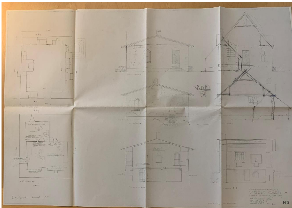
Utformningen före ombyggnaden 1969–70. Uppmätningar Per-Erik Nilsson 1968, GMA.
