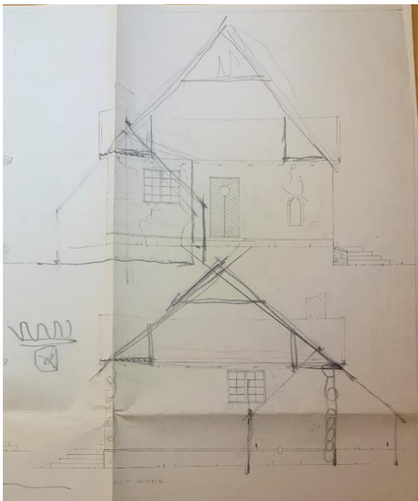
Uppmätningssritning en använd som skissunderlag för att pröva en högre takvinkel, sannolikt av Per-Erik Nilsson 1968, GMA.
