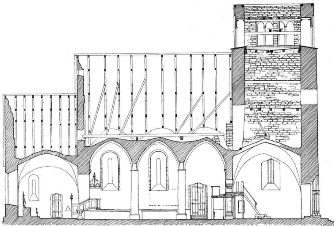
Längdsektion mot söder. Uppmätning Sten Wennerström och Adolf Niklasson 1921. Efter Sveriges Kyrkor volym 42, Gotland band II (1935).
