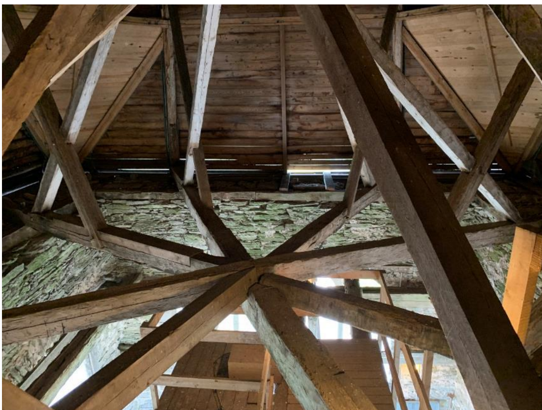
Tornhuvens bärande bjälklag mot norr. Foto JL 2021.
