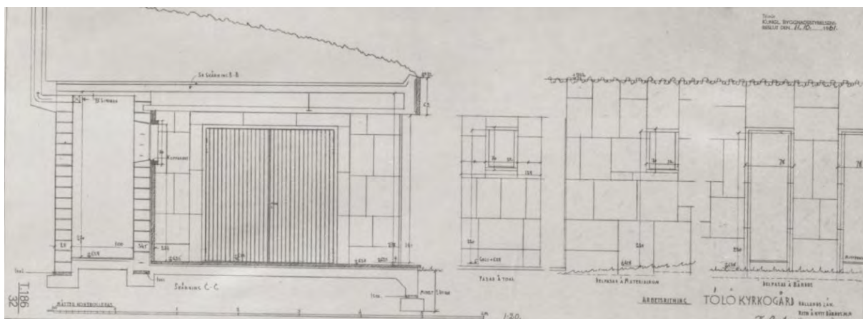
Sektion och fasader. Kaj Christensen, 1961. Källa: ATA/RAÄ
