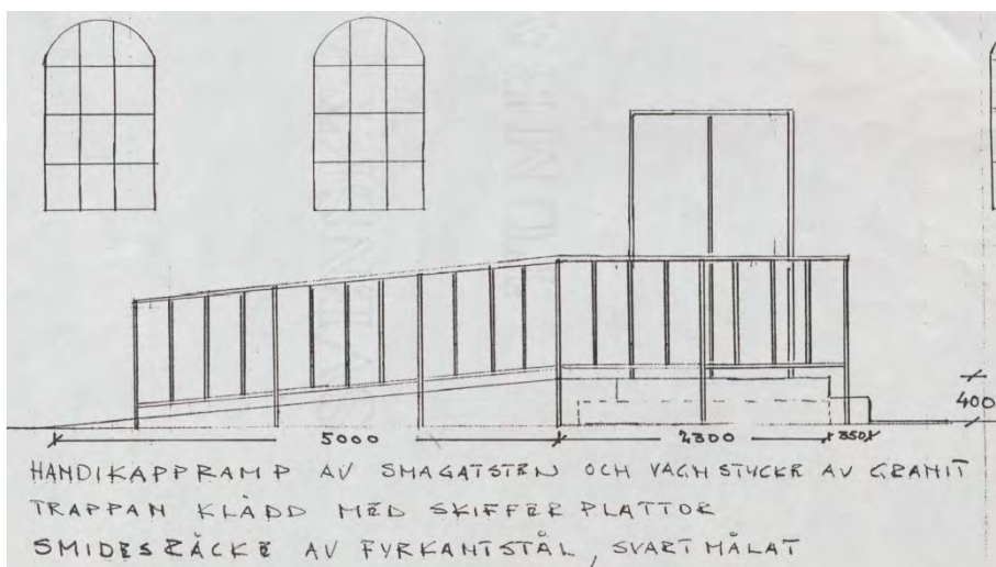
Skiss för handikappramp, 1992. Källa: ATA/RAÄ
