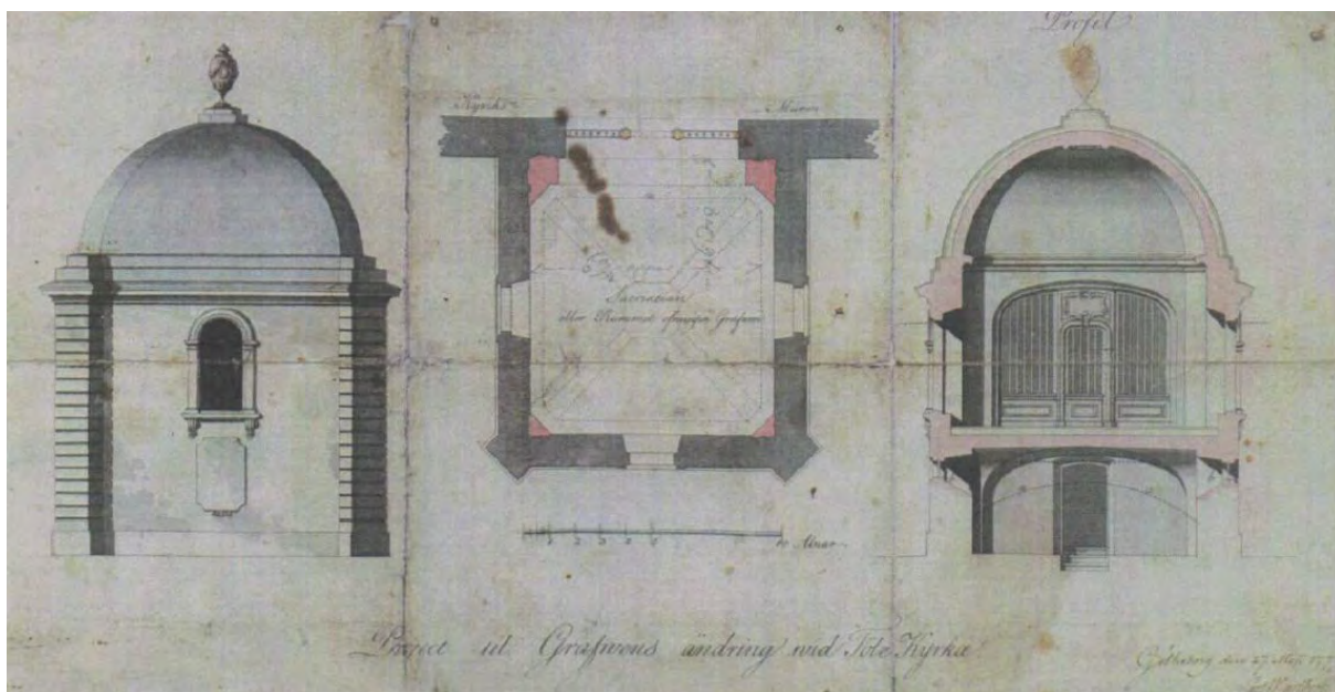
Ritning över gravkoret från år 1777, signerad Carl Wilhelm Carlberg. Källa: "Sahlgrenska/Silfverschiöldska gravkoret vid Tölö kyrka. Rapport över restaureringen år 2010", Kungsbacka kommun. Rapporten finns hos ATA/RAÄ
