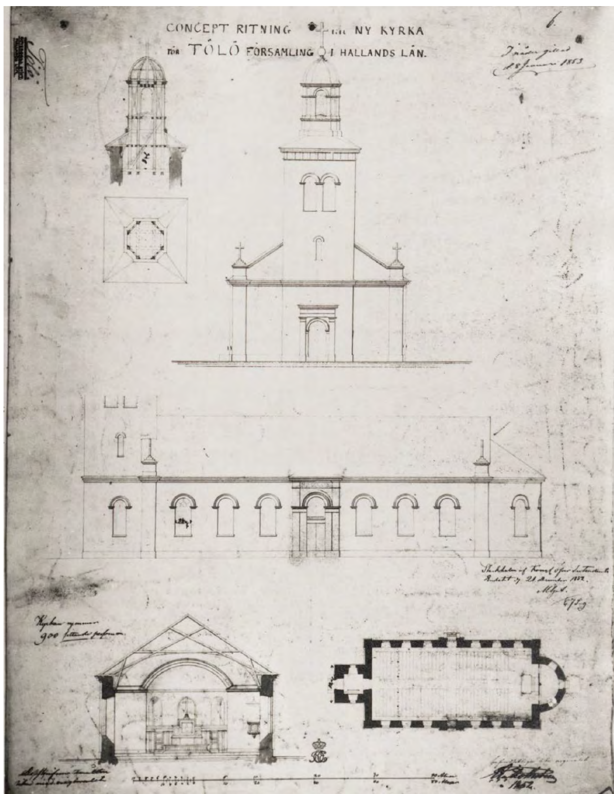
Ritning från år 1852, godkänd 1853. Källa: ATA/RAÄ.
