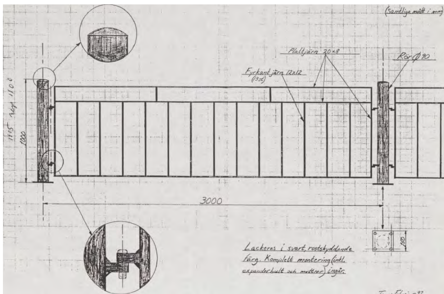
Utformning smidesräcke, 1992. Källa: ATA/RAÄ
