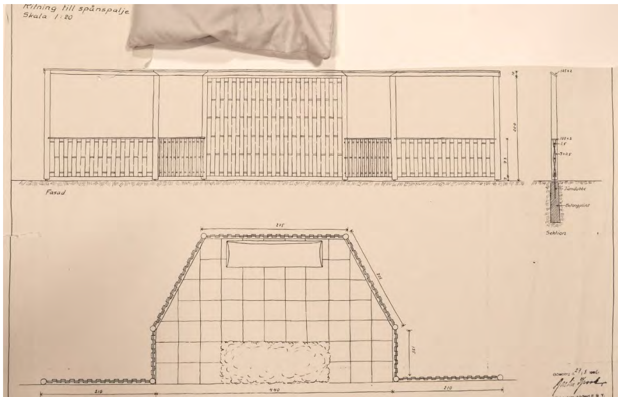
Ritning till spånspalje. Martin Krook, 27/8 1957. Källa: Älvsåkers kyrkoarkiv/Landsarkivet i Lund.
