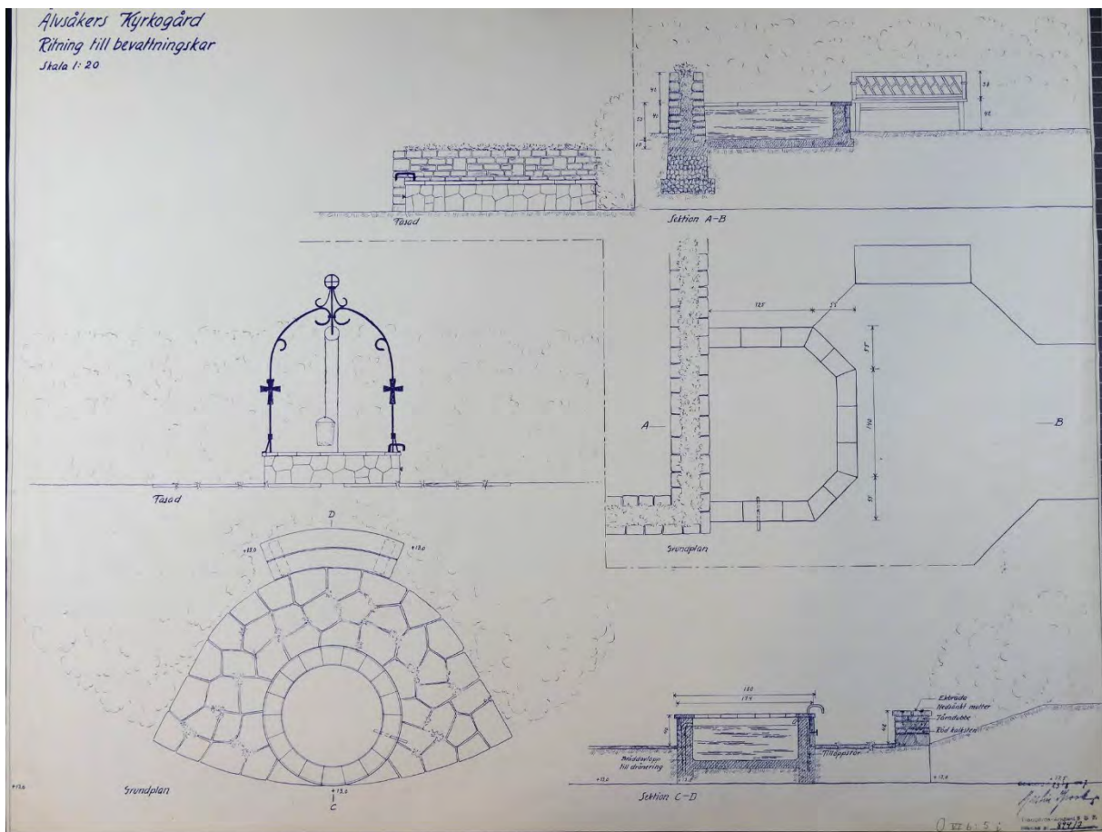
Ritning till bevarningskar, 23/8 1957. Martin Krook. Källa: Älvsåkers kyrkoarkiv/Landsarkivet i Lund.
