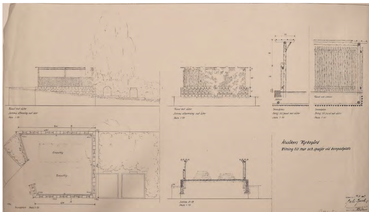
Ritning till mur och spaljär vid kompostplats. Martin Krook, 22/8 1957. Källa: Älvsåkers kyrkoarkiv/Landsarkivet i Lund.
