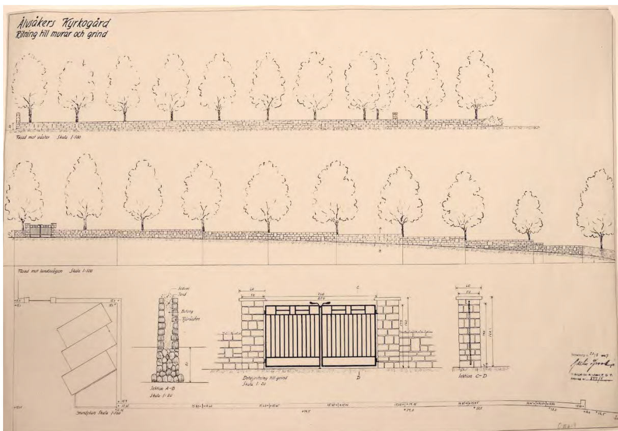
Ritning till murar och grind. Martin Krook, 23/8 1957. Källa: Älvsåkers kyrkoarkiv/Landsarkivet i Lund.
