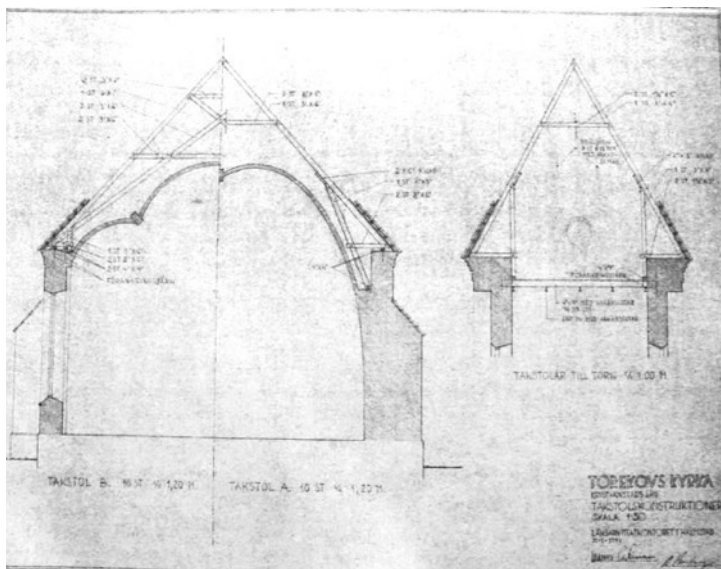
Takstolar över långhuset (två typer) samt tornet, ritn 1950
