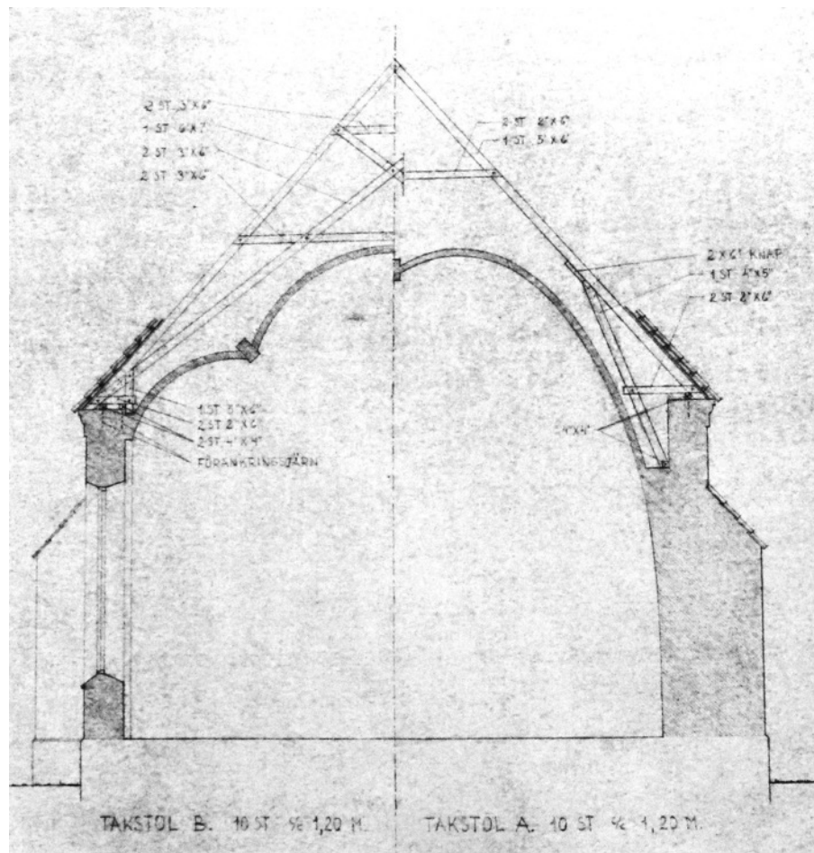
Carlmans tvärsektioner med tegelvalv och takstolar 1950
