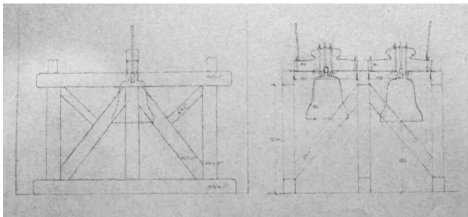
Klockbocken, ritn 1950
