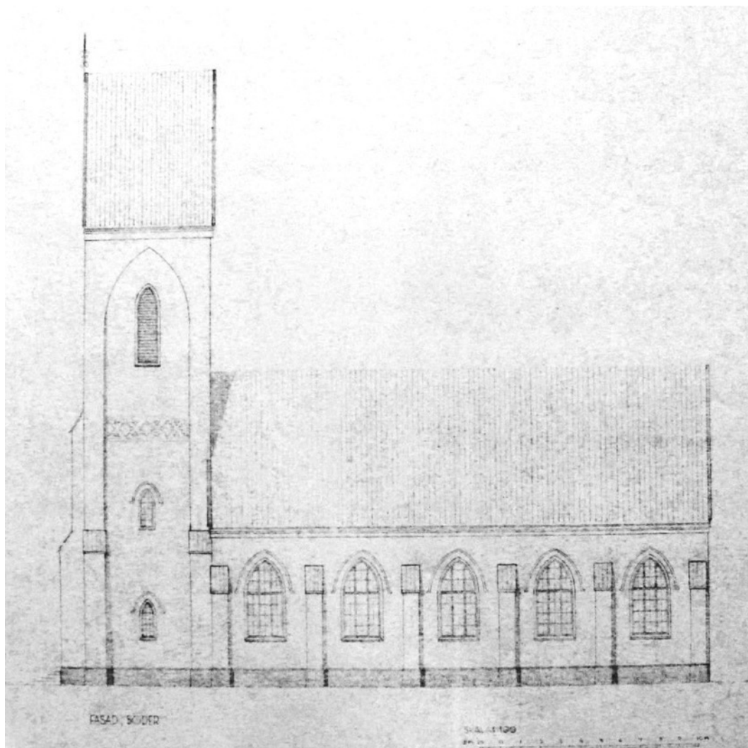
Carlmans sydfasad 1950
