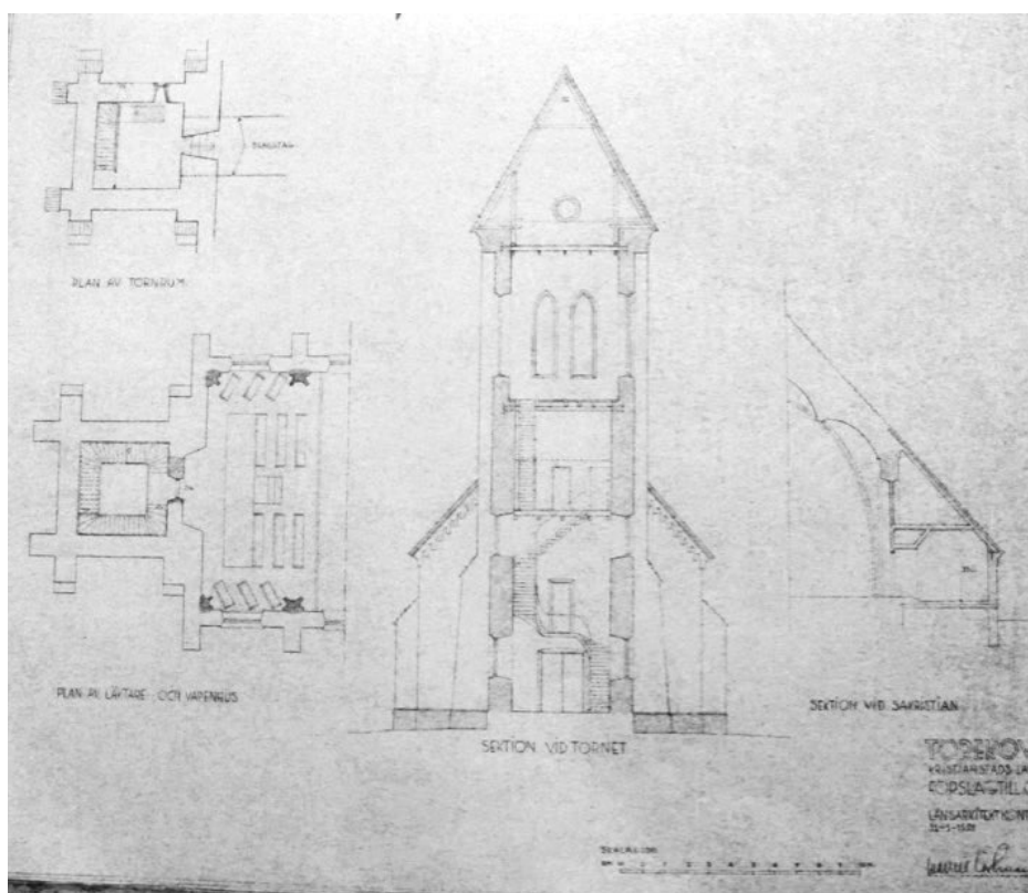
Bjälklag och takstol i tornet och sakristian, ritn 1950
