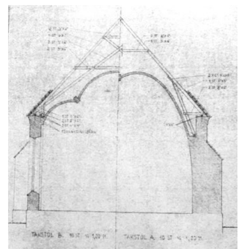
Tvärsektioner
