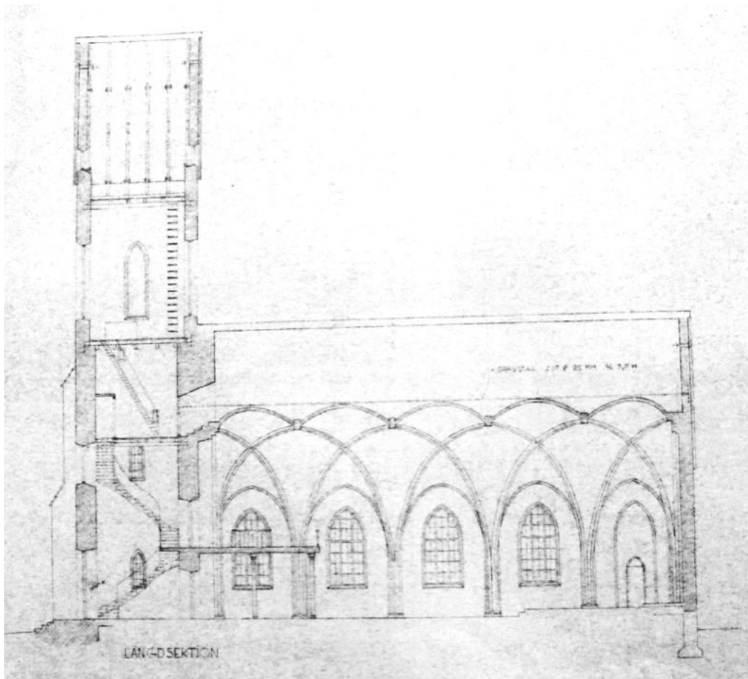
Carlman's längdsektion 1950
