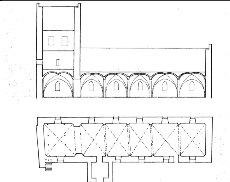
Längdsektion och plan av den senmedeltida kyrkan, skala 1:600
