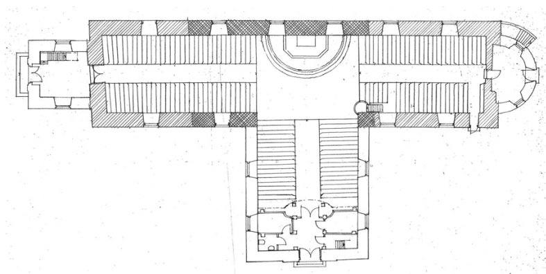
Plan av Västra Karups kyrka, skala 1:600
