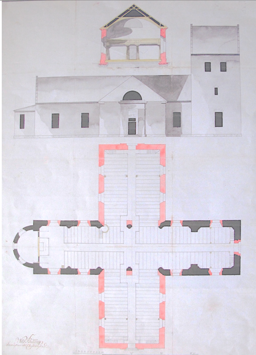
Plan, fasad och sektion till Västra Karups kyrka, Nils Billing, murmästare uti Christianstad 1803 (Riksarkivet)
