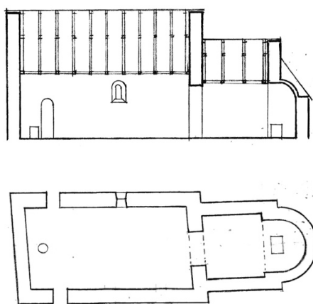
Längdsektion och plan av 1100-talskyrkan, skala 1:600 eventuella fönster på sydsidan och i koret är obekanta
