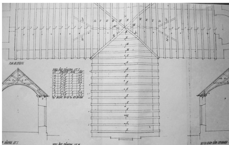
Takstolsplan 1950
