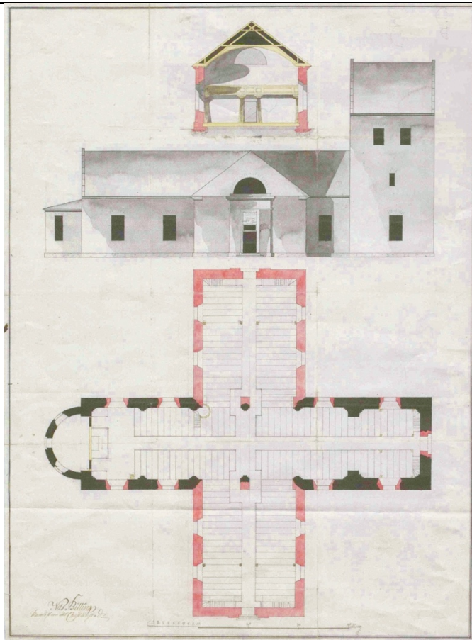
Förslag till tillbyggnader mot norr och söder, Billing 1803
