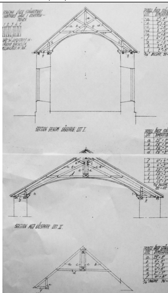
Takstolstyper 1950
