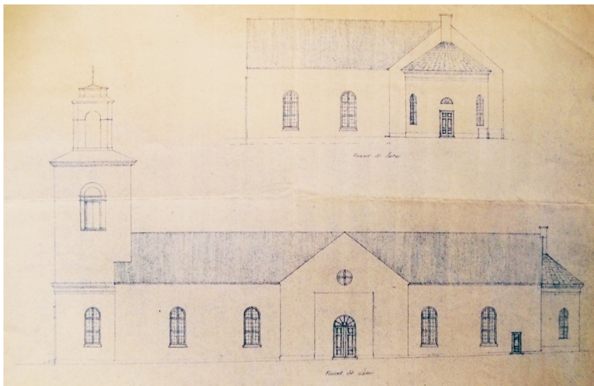
Fasader 1990, Thorsten Davidsson
