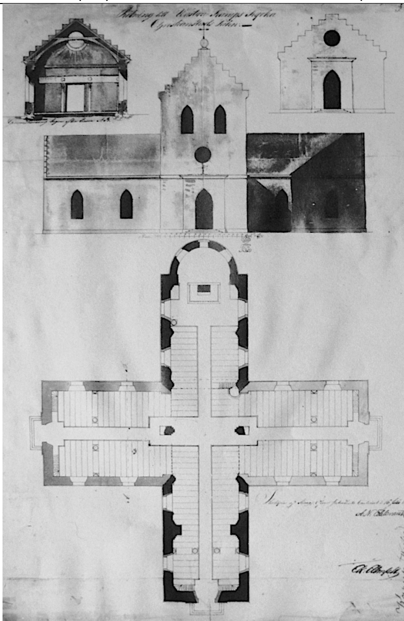
Ritning till Västra Karups kyrka i Christianstads län, plan. Fasader,sektion, Axel Almfelt, godk av överint.ämb. 16 juli 1805 (ATA)
