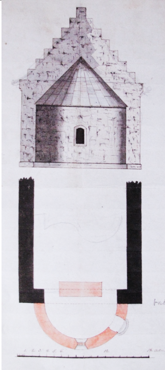
Tillbyggnad av Västra Karups kyrka. Plan och fasad av koret och sakristian, osignerad 1787 (Riksarkivet)
