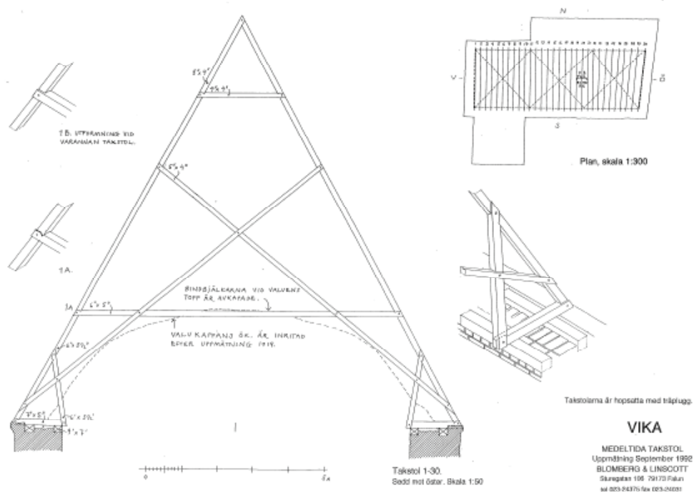
Uppmåtningsritningar hämtade ur Medeltida takstolar i Dalarnas kyrkor. Blomberg och Linscott 1993.
