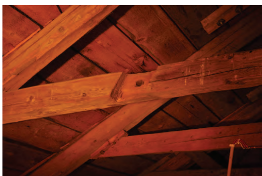
Många hanbjälkar har urtagat på bild. Foto: Daniel Eriksson.
