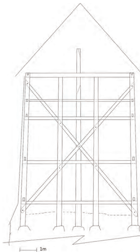
Figur 20. Principskiss av klockstapelns stomme sedd från öster.
