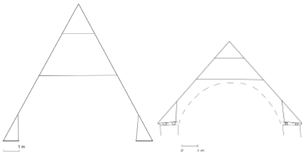
Munktorps kyrkas långhus. Schematisk skiss som visar några medeltida delar i långhusets taklag.
