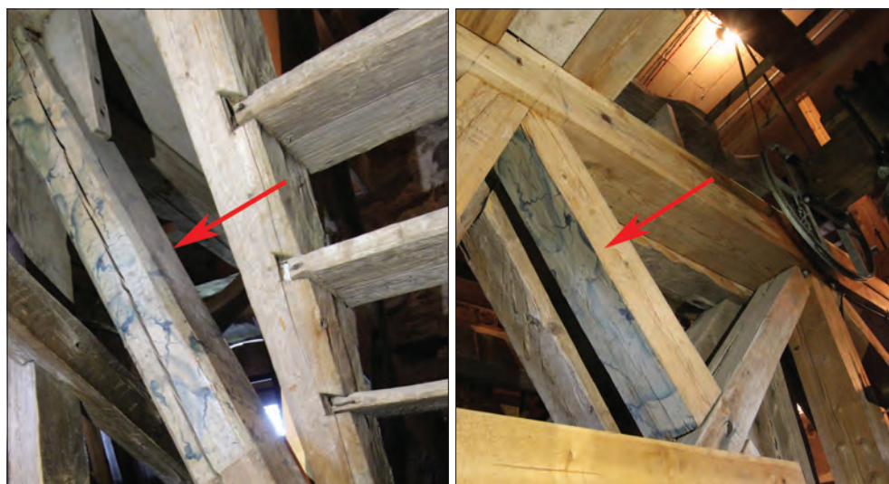
Figur 17. Marmoreringsmålade bjälkar finns i bockkonstruktionen i klockvåningen. Eventuellt kan de komma från någon tidigare läktaruppgögnad från kyrkan. De är inte medeltida, men åldern har inte utretts.
