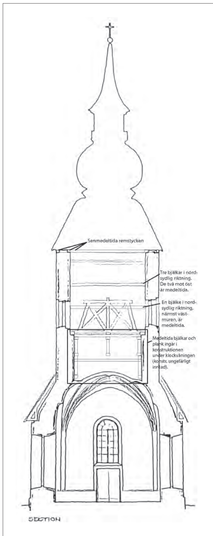
Figur 3. Sektion, sedd från väster, genom tornet med markeringar var återanvänt medeltida virke förekommer. Sektionen är upprättad av Göran Berglund Arkitektkontor AB 1991 i samband med en yttre och inre renovering (Dalarnas museums topografiska arkiv).
