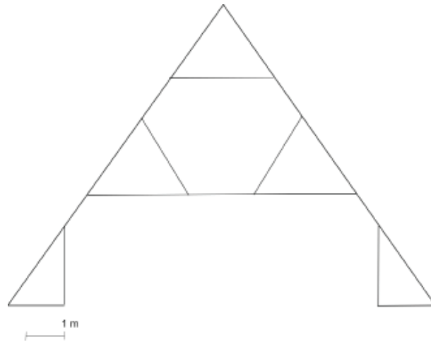
Del av den medeltida takstolskonstionen, långstolen är inte skissad.
