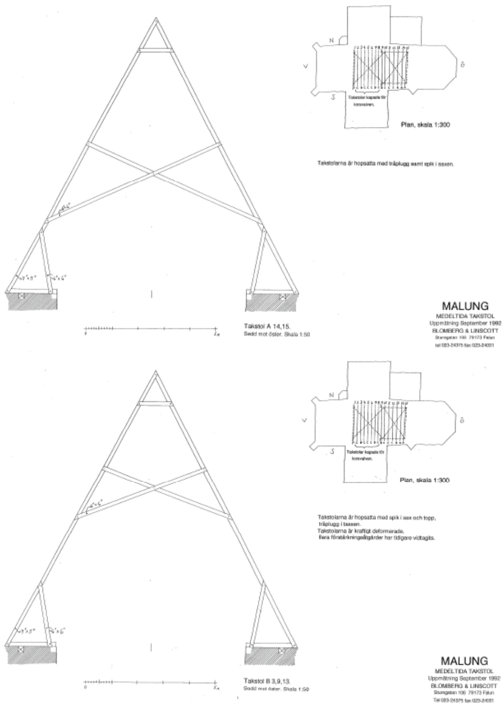
Uppmättningsritningar hämtade ur Medeltida takstolar i Dalarnas kyrkor. Blomberg och Linscott 1993.
