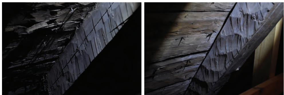
Sprättäljning räkt respektive diagonalt. Foton: Daniel Eriksson.
