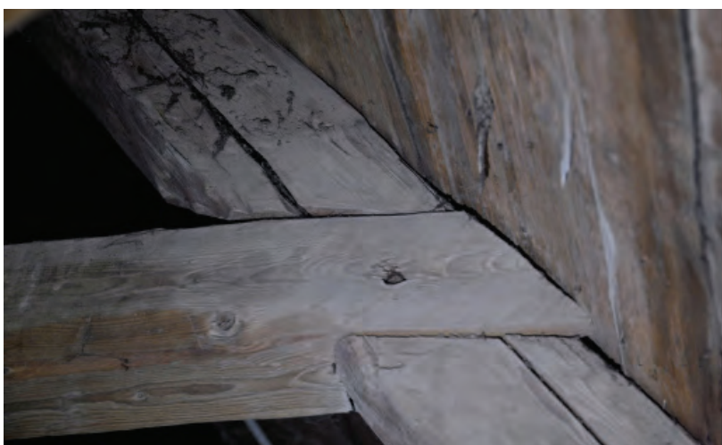
Rak bladning med spik respektive bladning halvt i halvt med spik. Foto: Daniel Eriksson.
