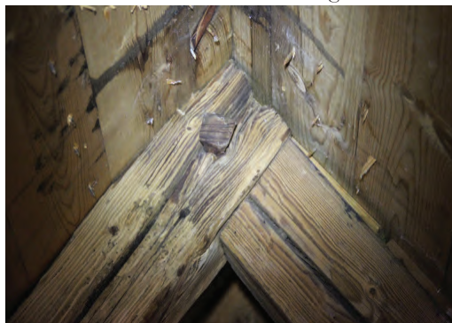
Inock är högbenen troligen sammanfogade genom tapp och slits.
