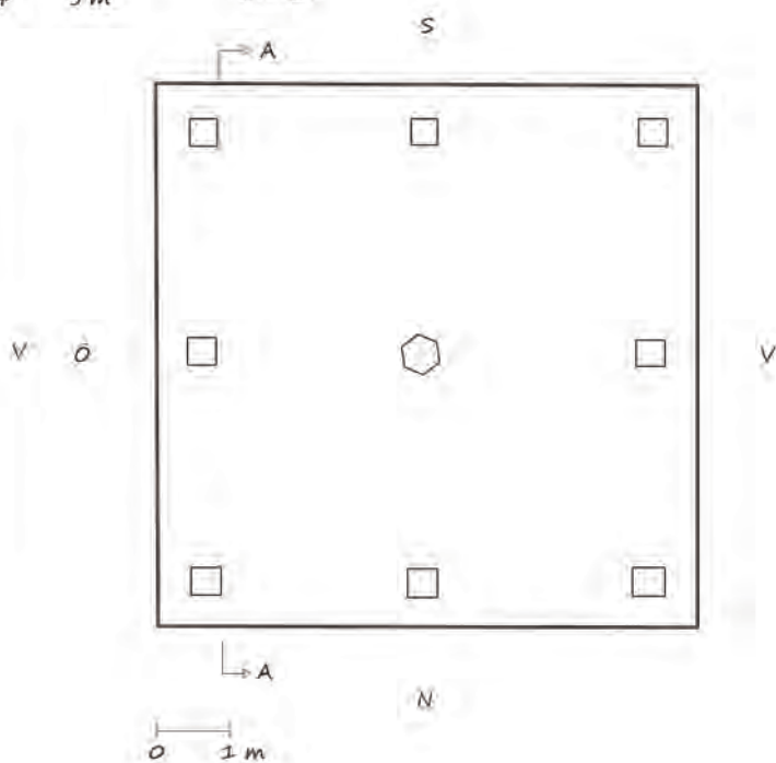
Plan genom klockstapelns nedre del.
