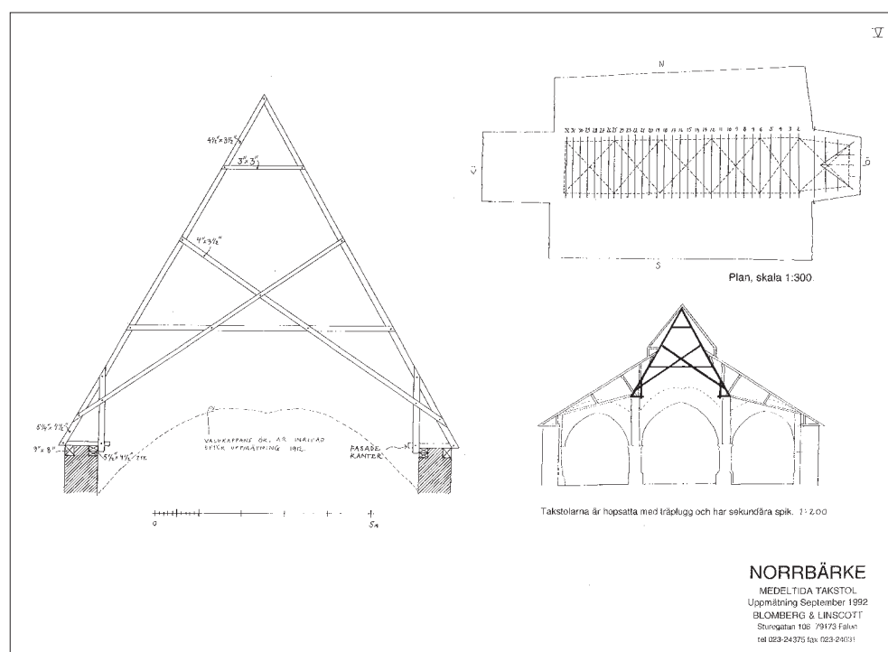
Figur 16. Uppmätningsskizningar från Norrbärke kyrka av Blomberg och Linscott 1992.
