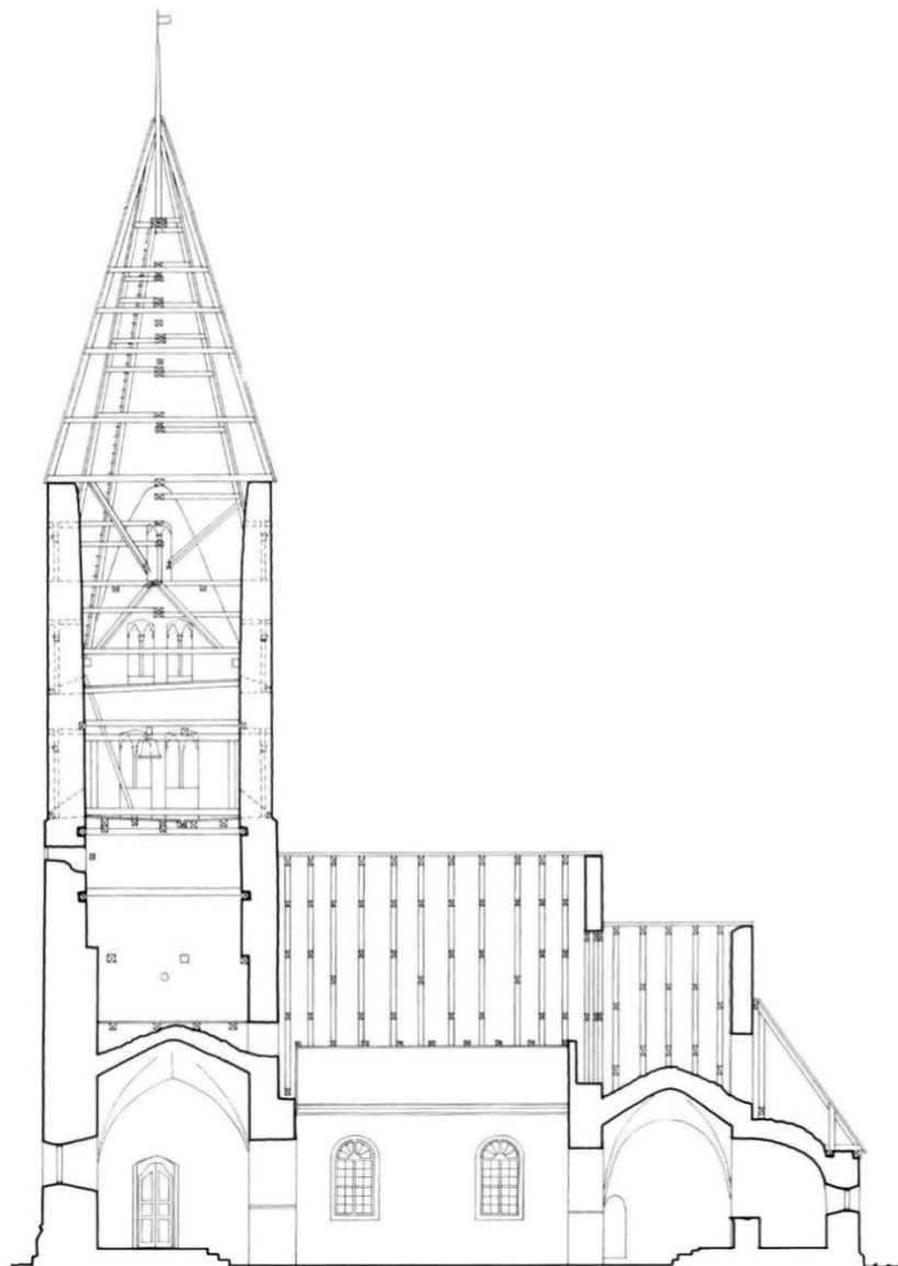
SKÄRNING A-A.
