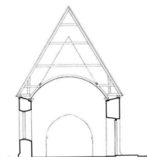
SKÄRNING B-B.
