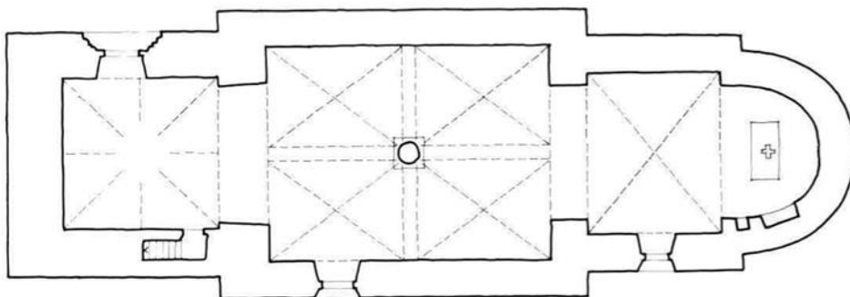
Kyrkans plan före 1839-40. Fönster och annan inredning än högaltaret ej markerade. Möjligen var den ursprungliga triumfbågen smalare. Rekonstruktion Erland Lagerlöf och Gunnar Wirén 1982. Efter Sveriges Kyrkor, Gotland VIII:2 , volym 191.
