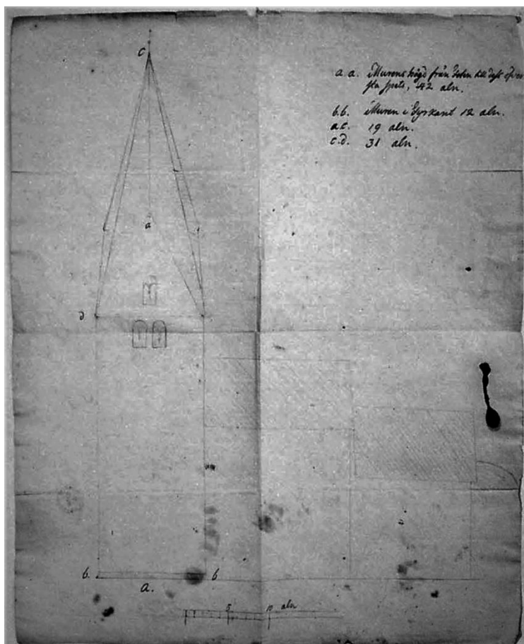
Kyrkans fasad mot söder. Uppmätning 1780, utförd som underlag för förslag till nytt tornkrön. Efter Sveriges Kyrkor, Gotland VIII:2, volym 191.
