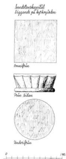
Bevarade delar av den 1839–40 rivna kolonnen. Uppmätning John Söderberg 1943. Sveriges Kyrkor, Gotland VIII:2, volym 191. Foto JL 2019-2020.
