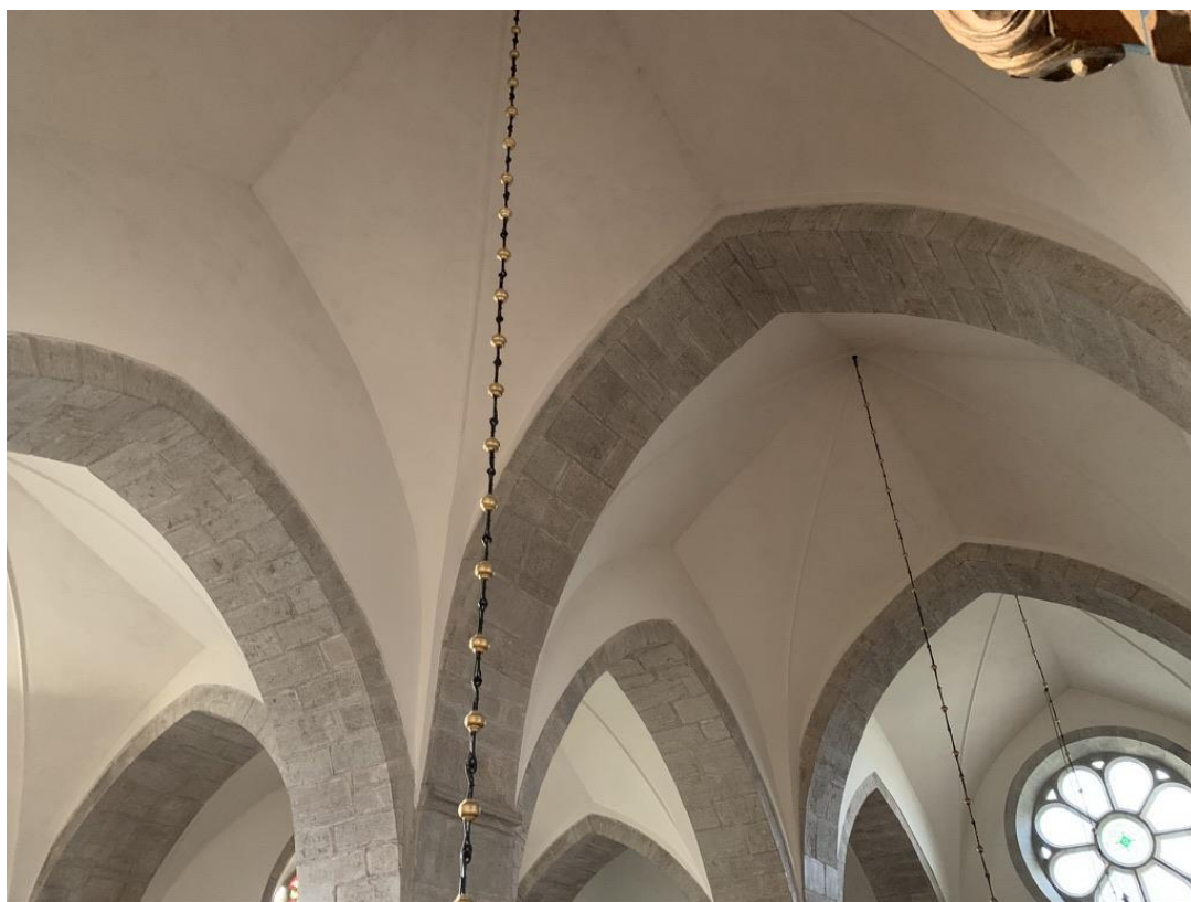
Valven i långhuset, sedda snett underifrån mot sydväst. Observera att den östligaste bågen längst till vänster ligger något lägre i förhållande till valvet än de båda andra. Det och andra detaljer talar för att långhuset byggdes i två etapper. Foto JL 2019.
