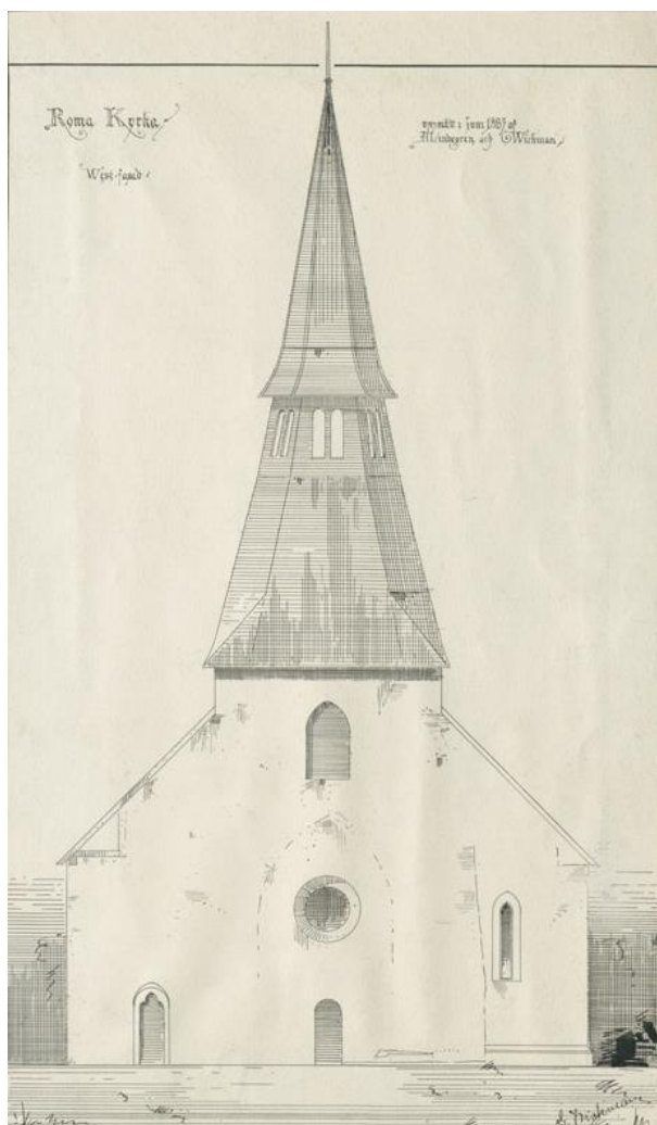
Västfasaden 1883 och omkring 1920. Observera rundfönstrets och mitskeppsportalens äldre utformning till vänster. Uppmätning Agi Lindegren och Gustaf Wickman 1883 resp. efter Sveriges Kyrkor, Gotland I:5, volym 35.
