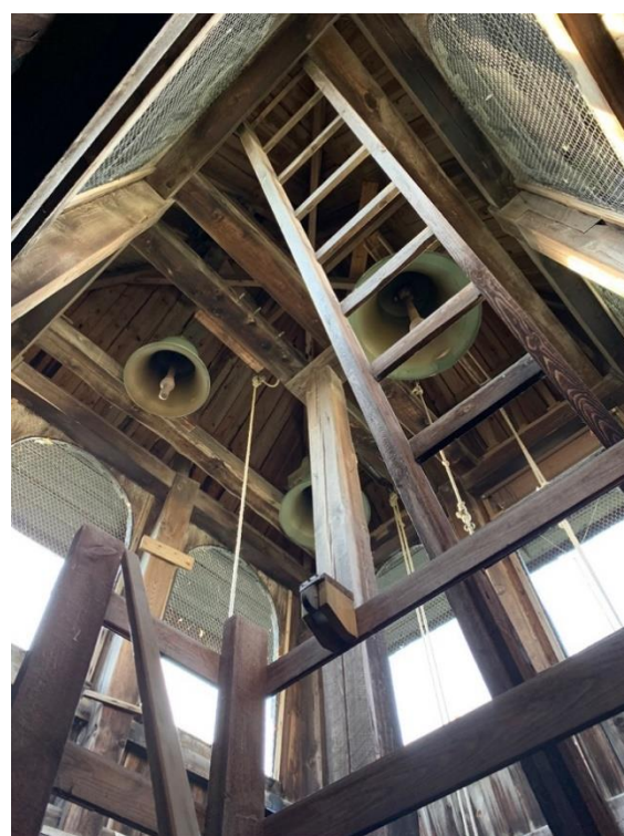
Svenskbystapeln. Byggt 1939 för att rymma de klockor som tagits med från Gammalsvenskby i Ukraina. Drivande för stapelns tillkomst var biskop Torsten Ysander. Erik Lundberg ritade stapeln efter medeltida förebilder i Danmark och Sydsverige. Den restes av Reinhold Lydahl, Etelhem. Foto JL 2017 (exteriör) och 2019 (interiör).
