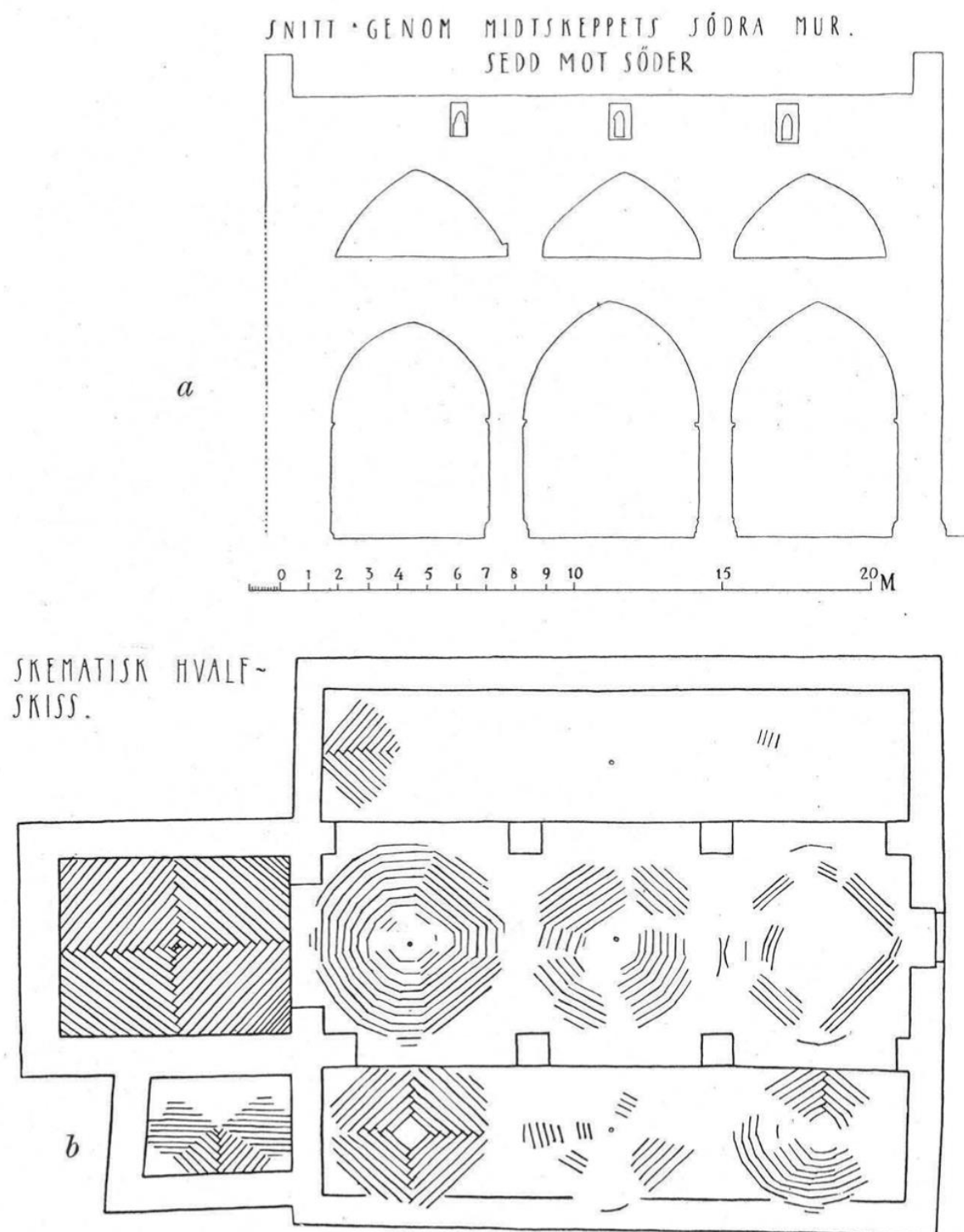
Mittskeppets södra mur och valvplan (koret i öster åt vänster). Uppmätning omkring 1920. Efter Sveriges Kyrkor, Gotland I:5, volym 35 (1931).
