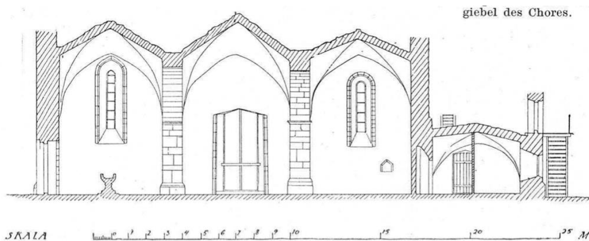
Längdsektion genom norra sidoskeppet och sakristian. Uppmätning omkring 1920. Efter Sveriges Kyrkor, Gotland I:5, volym 35 (1931).
