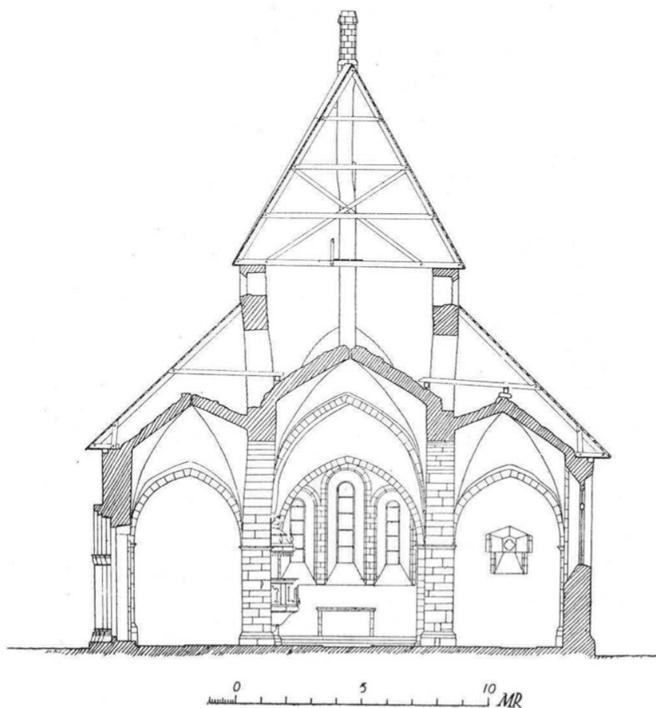
Tvärsektion mot öster. Uppmätning omkring 1920. Efter Sveriges Kyrkor, Gotland I:5, volym 35 (1931).
