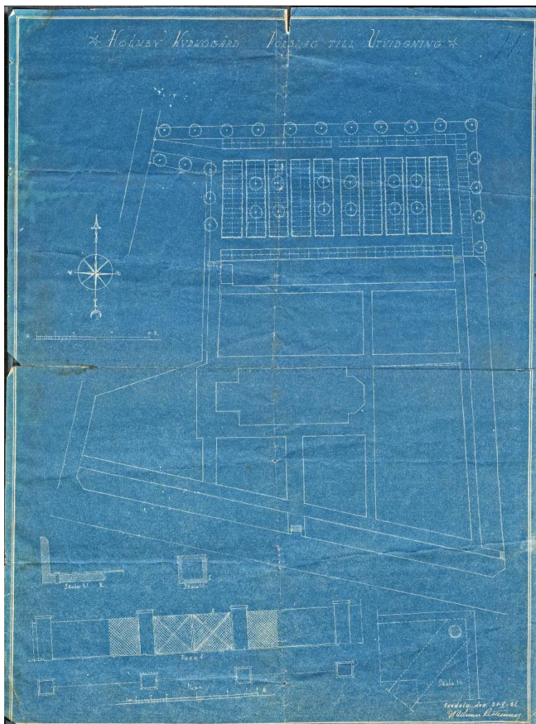
Blåkopia av ritning över den nyare delen av kyrkogården i Holmby. Ritningen är daterad den 28 maj 1926. Källa: Kyrkoarkivet.
