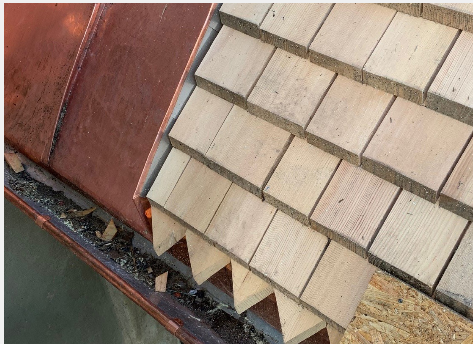
Vid takfoten avslutas taket med spetsiga spån.
