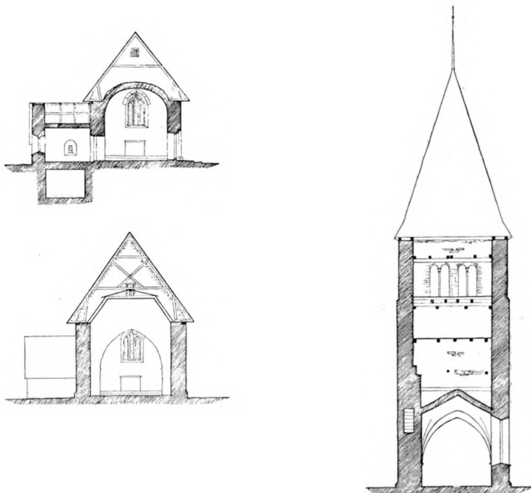
Sektioner av kor och sakristia mot öster, långhuset mot öster samt tornet mot öster. Tornhuvens konstruktion ej utritad. Uppmätning av Erik Persson och Karl Karlström 1928. Efter Sveriges Kyrkor (68), Gotland band IV:3 (1952).
