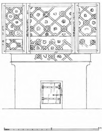
Altarets baksida med målning på altarskåpets utsidor samt luckan för nischen i altaret. Uppmätning av Erik Persson och Karl Karlström 1928. Efter Sveriges Kyrkor (68), Gotland band IV:3 (1952).
