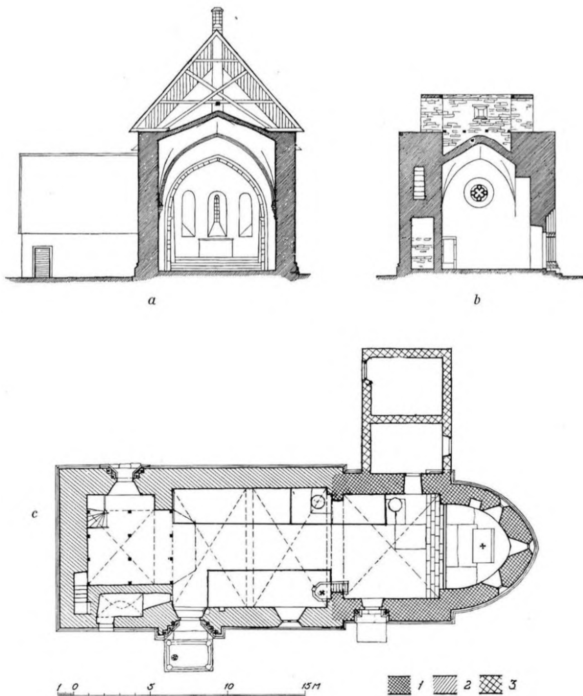
Tvärsektion genom långhuset mot öster och genom tornet mot väster (tak och tornhuv ej medtagna) samt plan. Uppmätning av K. J. Karlström och E. Persson 1928. Efter Sveriges Kyrkor, Gotland band III, volym 54 (1942). Byggnadsperioderna avser 1: 1200-talets början. – 2: 1200-talets slut. – 3: 1800–01. Vid restaureringen 1956–57 revs läktaren och avlägsnades kaminen. Passage är upptagen mellan sakristian och magasinet, som har innerväggar och i vars bortre del finns en bred trappa till övervåningen.
