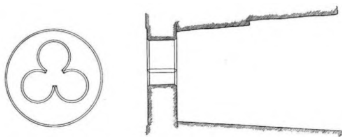
Fig. 119. Fönster i inclusorie-cellen åt kyrkorummet till. Skala 1:20. Fenster im Inclusorium gegen den Kirchenraum.
