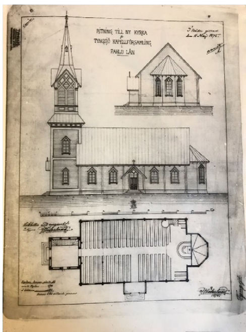
Ritning över Tyngsjö kyrka 1875, ATA.
