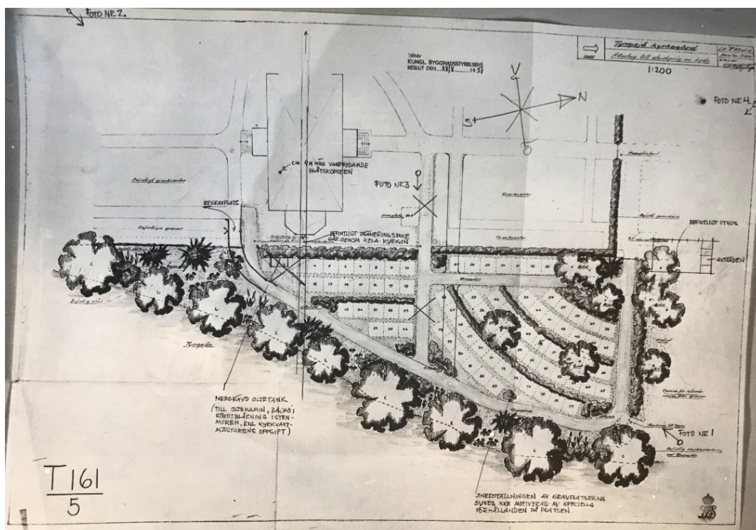
Ritning över kyrkogårdsutvidgning 1957, ATA.
