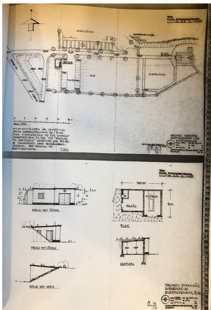
Ritning över bisättningsrum och parkering, Kommunernas konsultbyrå 1964, ATA.
