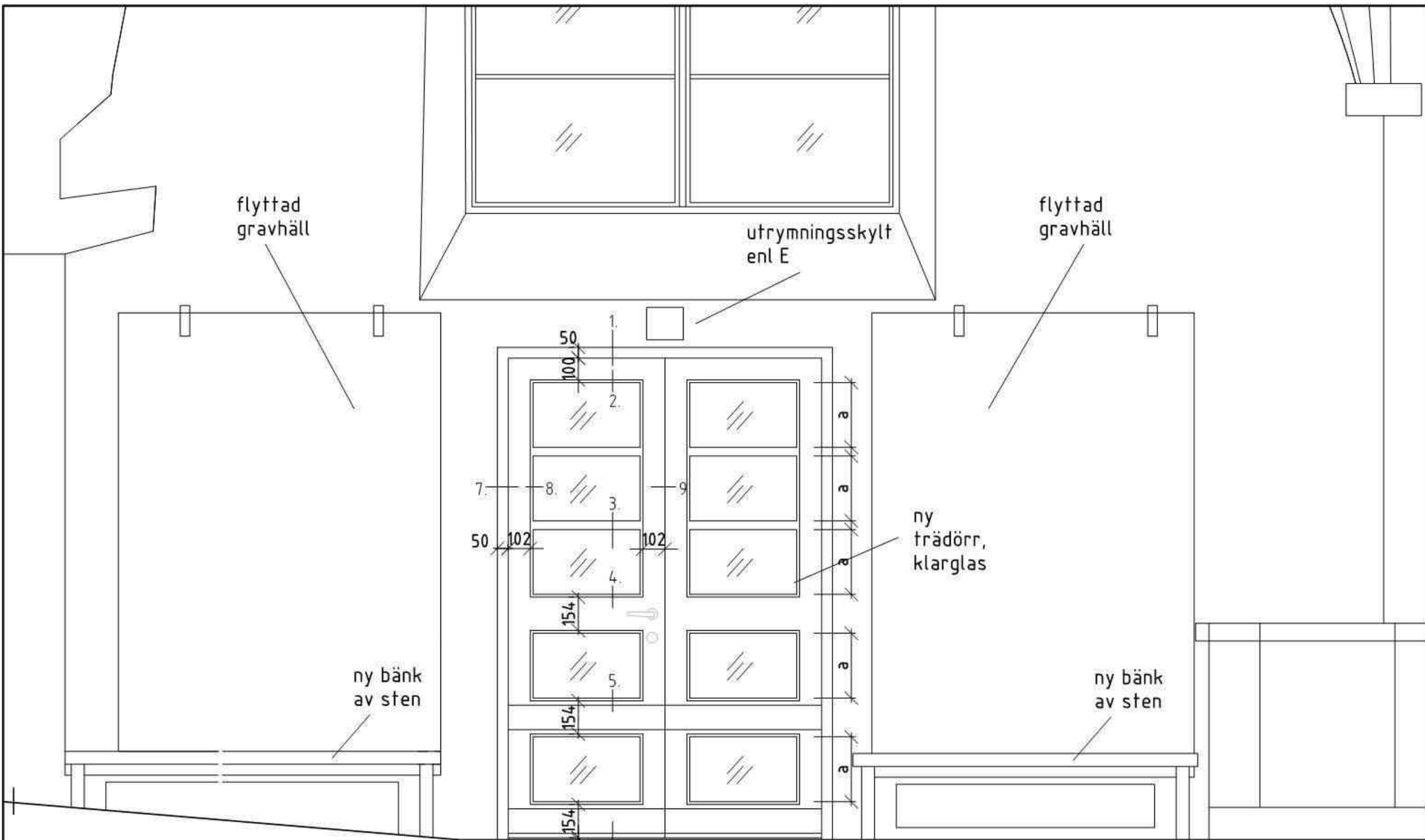
D12b - Kyrkorum - Elevation
