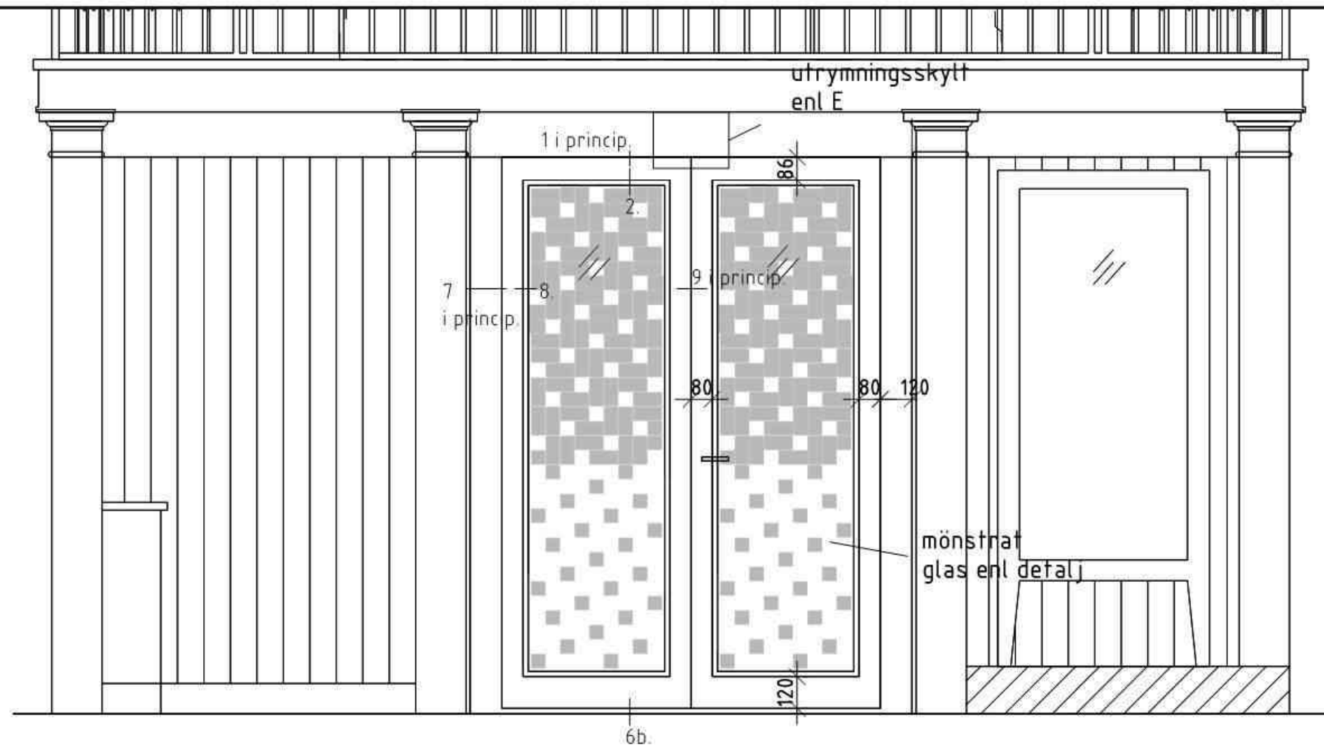
Förrum - Västra entrén 1:20 (A1)
