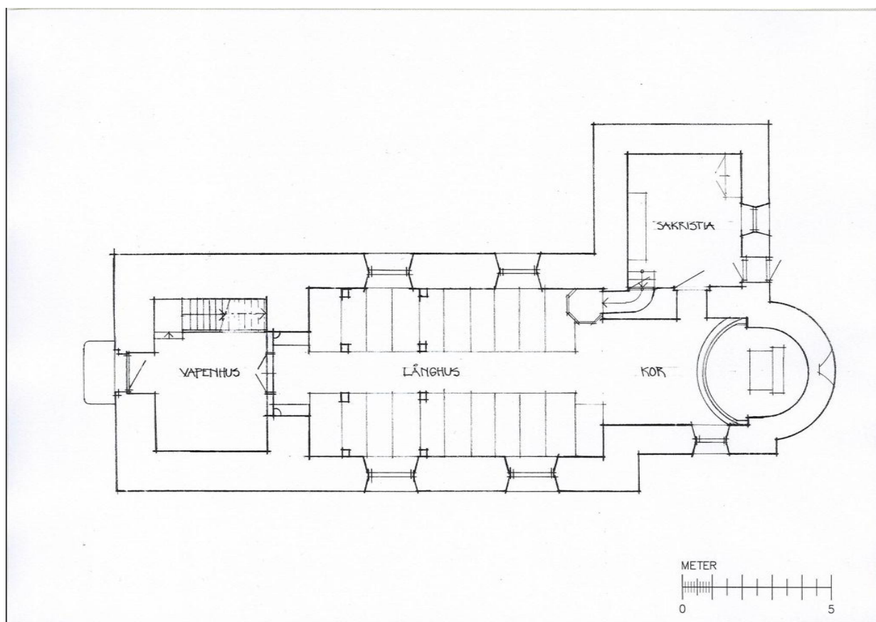
Bild 1: planritning, ur vård- och underhållsplan, ATRIO arkitektkontor 2005.
