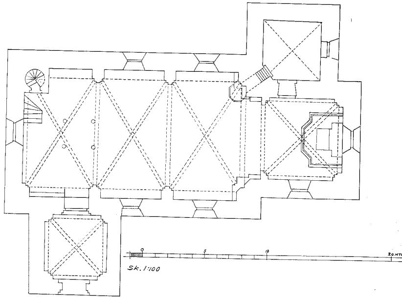
Börje kyrkas plan. Efter en uppmätning av Anders Roland 1911 (i Byggnadsstyrelsens arkiv).
