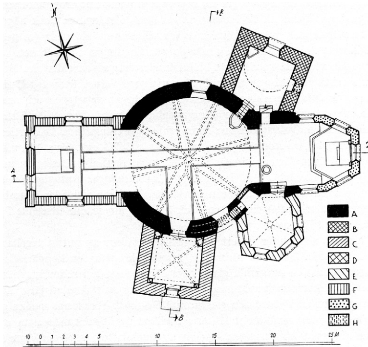
Plan av kyrkan mot norr. Uppmätt av John Söderberg 1948. Sveriges Kyrkor.
