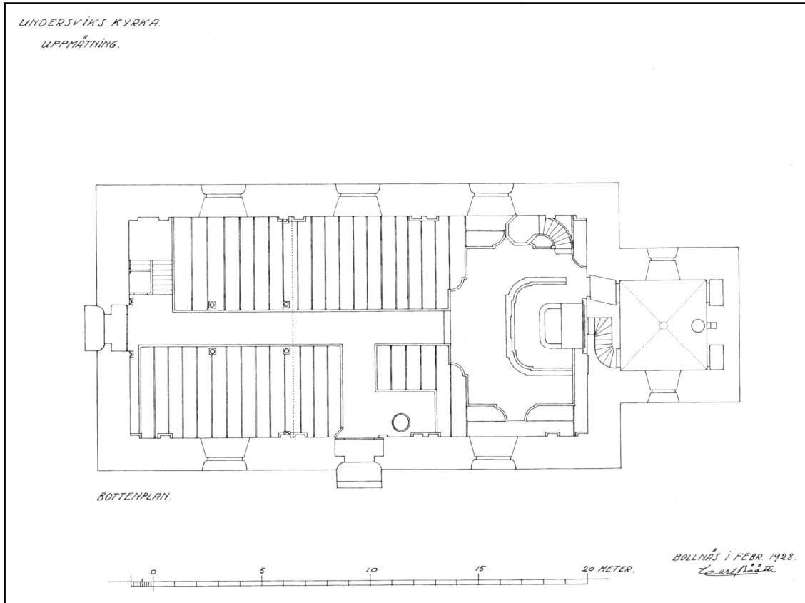
Ovan: Uppmättningsritning av Carl Bååth från 1928. Nedan: Carl Bååths ombyggnadsritning inför 1928 års renovering.
