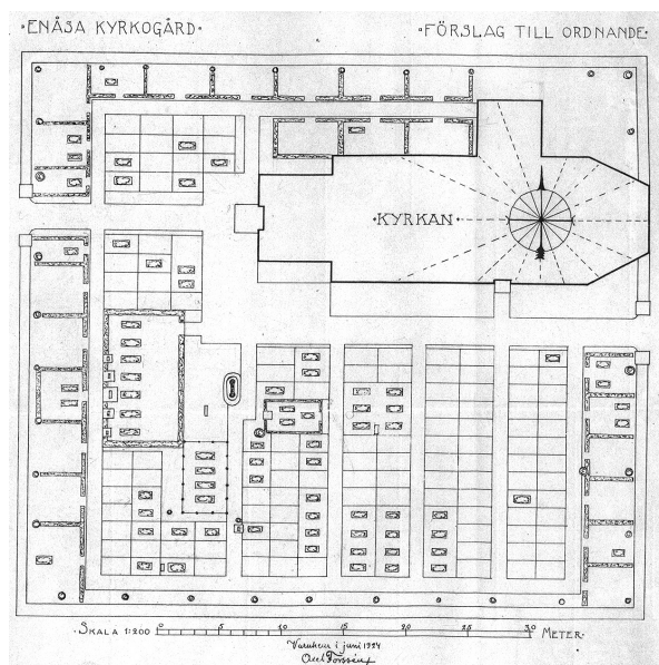
Ovan till vänster: Arkitekt Axel Forsséns uppmättningsritning från 1924. Ovan: Förslaget till ordnande av kyrkogården. Arkivhandlingar, ATA. Vänster: Foto taget av arkitekt Axel Forssén, möjligen inför det förslag till ordnande av kyrkogården han upprättade 1924. I det högruxna gräset på kyrkans sydsida kan ett antal be vuxna gravkullar skönjas. KALLA PÅ BILD.
